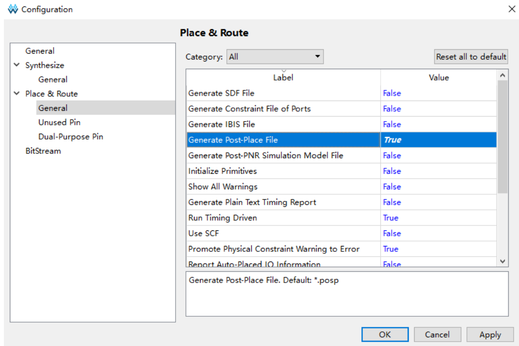
图 3-1 配置布局布线 Post-Place File 选项
