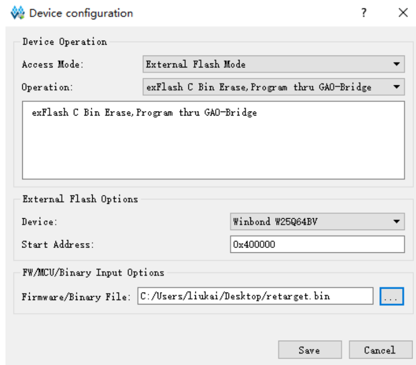
图 4-5 软件下载 Device configuration
