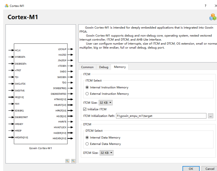
图 2-2 配置 ITCM Initialization
