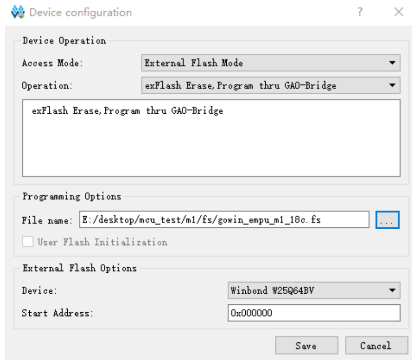
图 4-4 硬件下载 Device configuration
