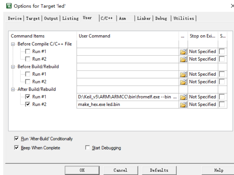
图 2-1 配置外部工具
