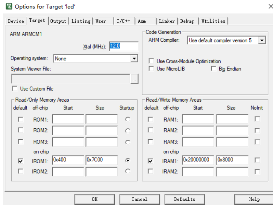
图 4-1 ROM 起始地址和容量配置
