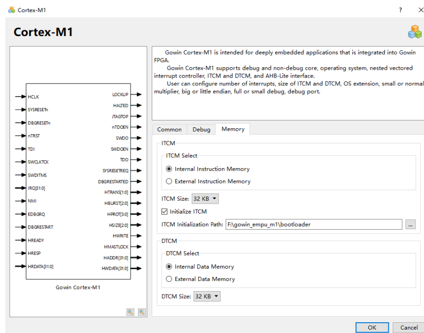
图 4-2 配置 ITCM Initialization Path 选项
