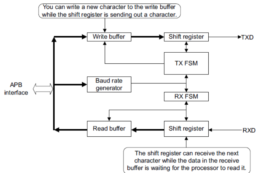
图 4-1 UART Buffering
