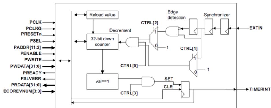
图 5-1 Timer
