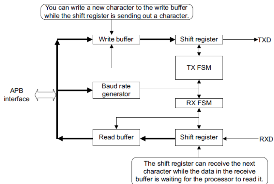
图 4-1 UART Buffering
