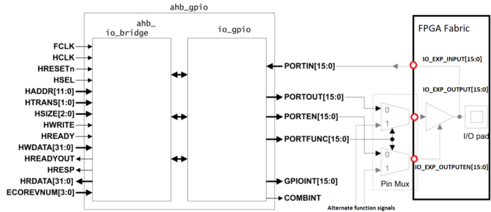
图 7-1 GPIO Block
