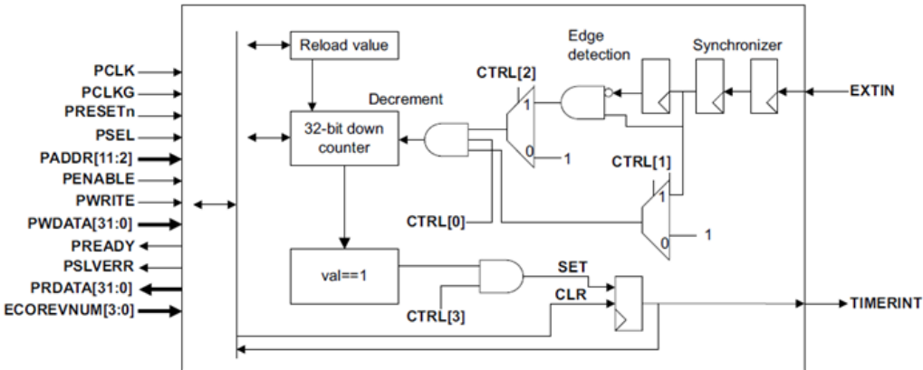
图 5-1 Timer
