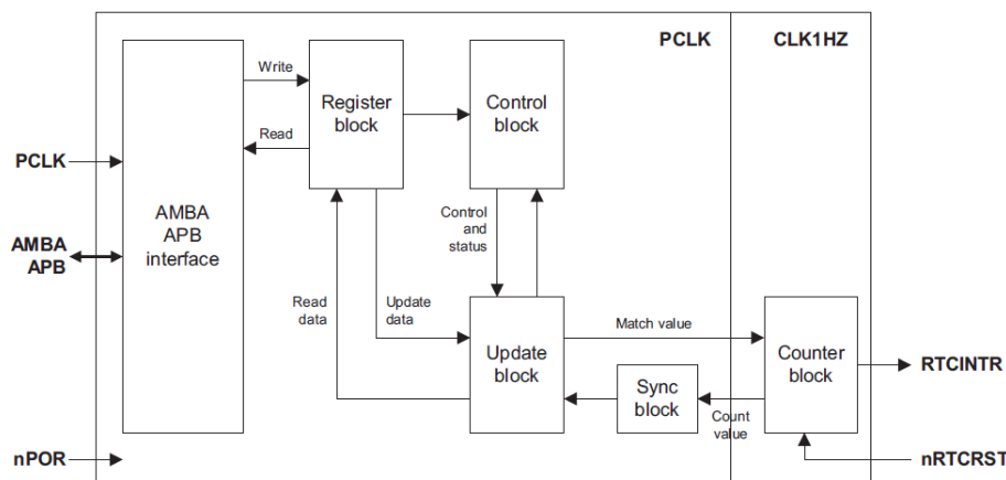
图 10-1 RTC Block
