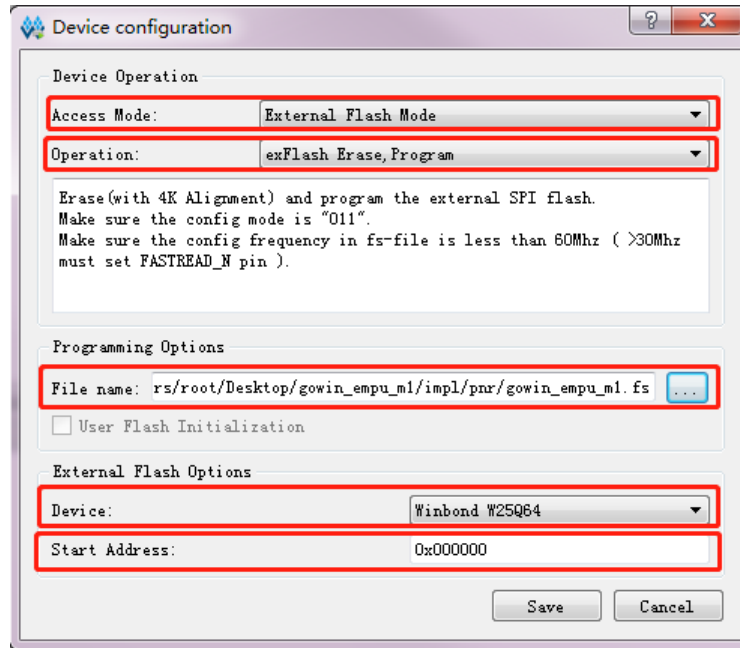
图 3-4 Configure Device
