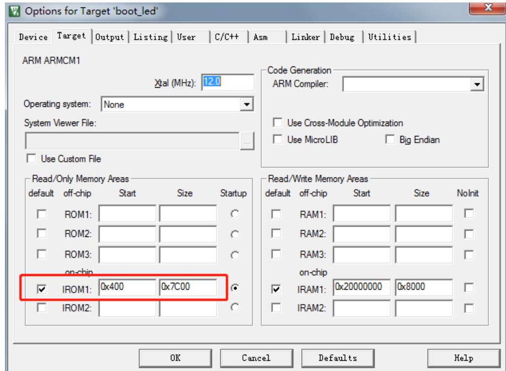
图 2-2 ROM 起始地址和 Size 配置
