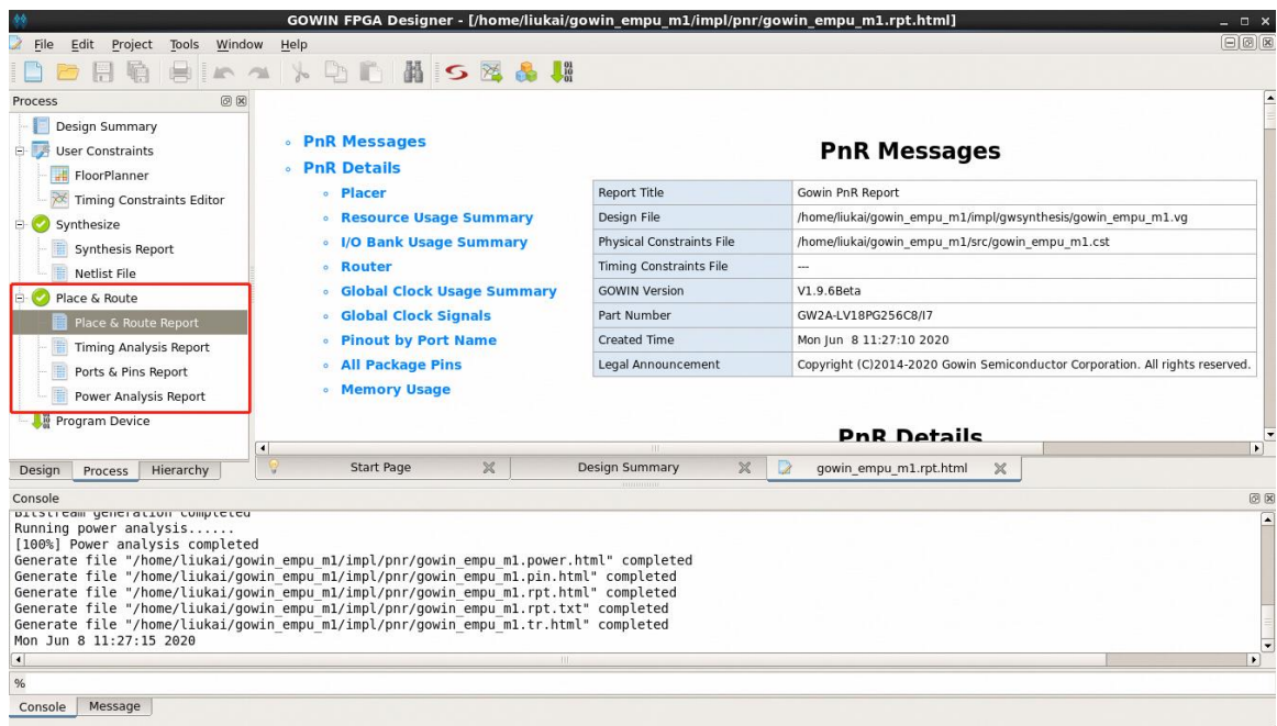
图 3-3 布局布线
