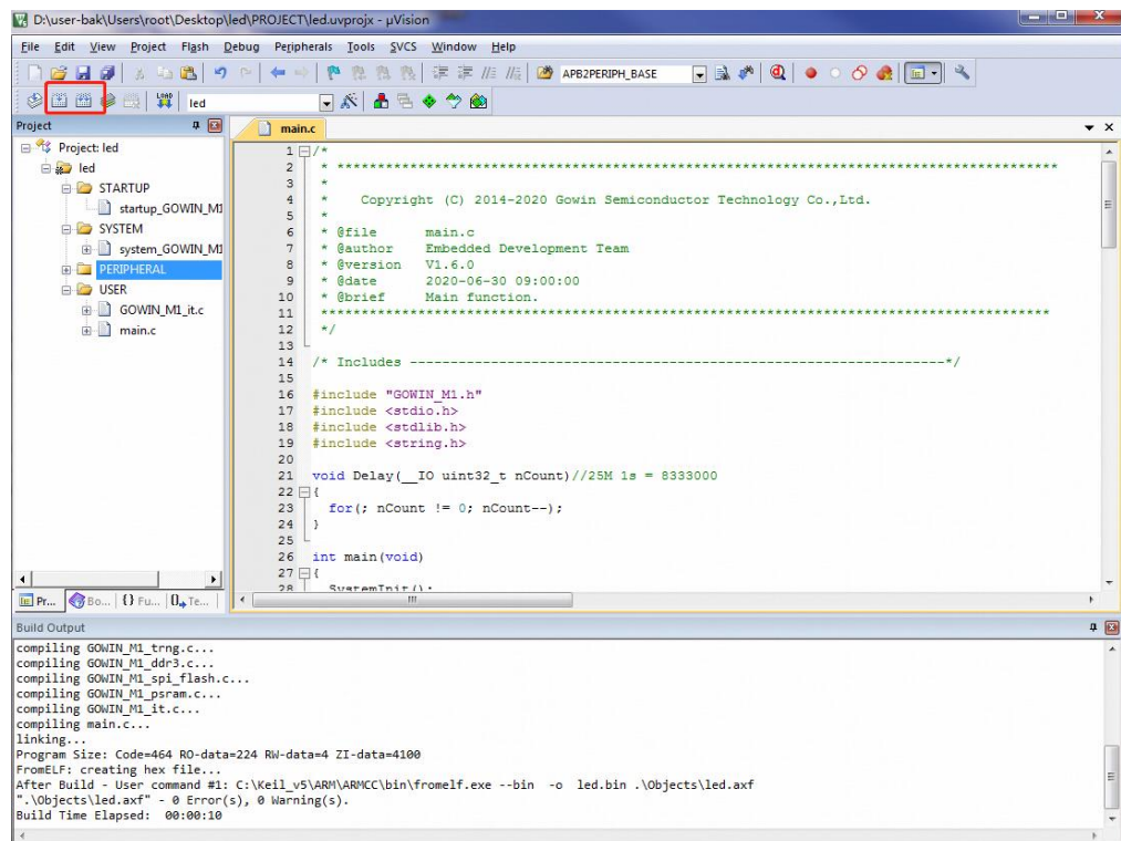
图 2-3 编译
