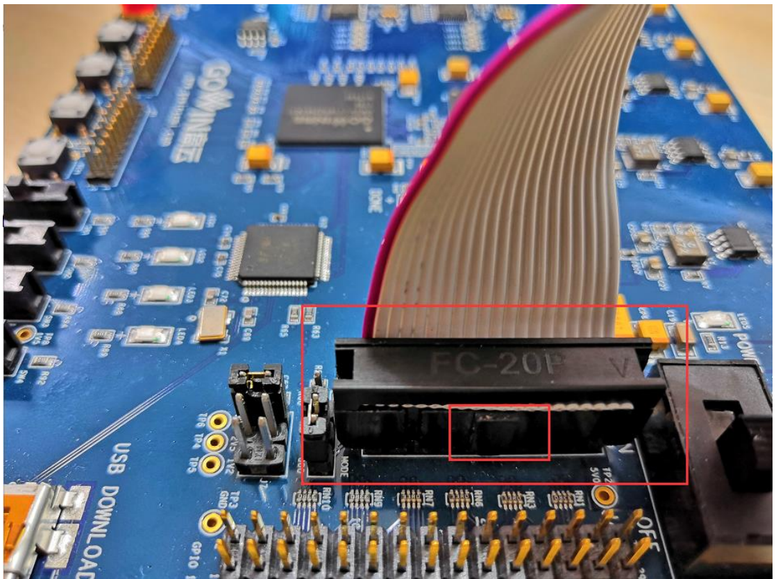
图 1-10 仿真器连接
