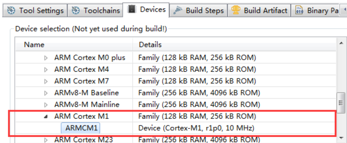
图 2-9 配置 Devices
