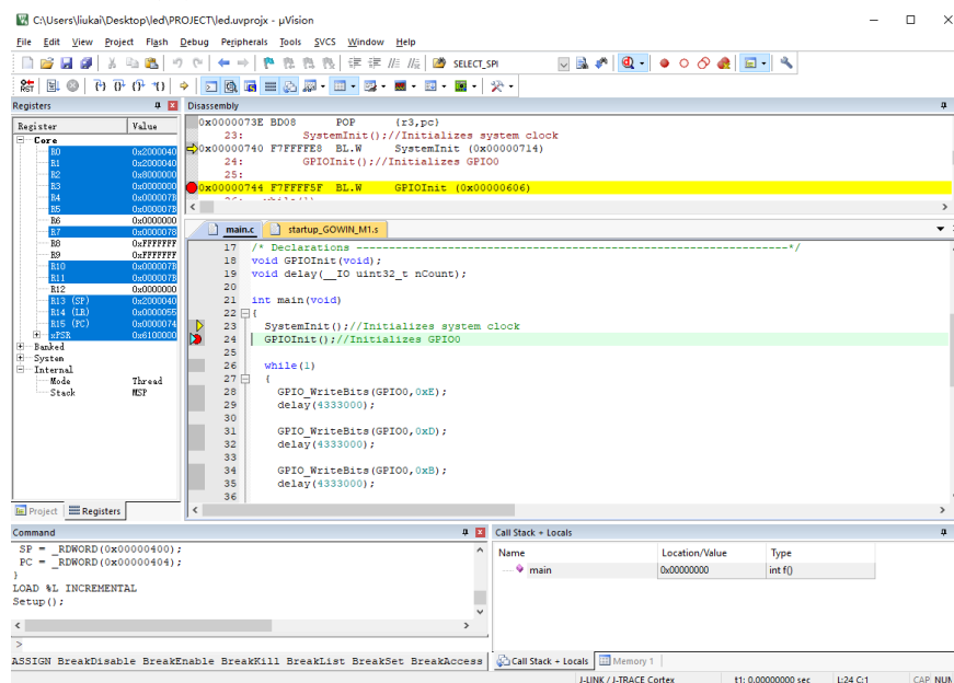
图 1-12 启动调试
