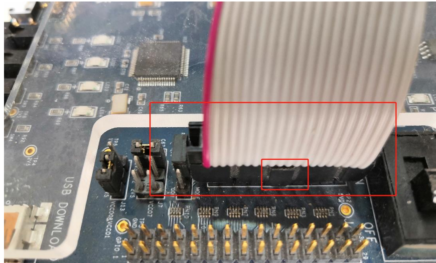
图 1-11 仿真器连接
