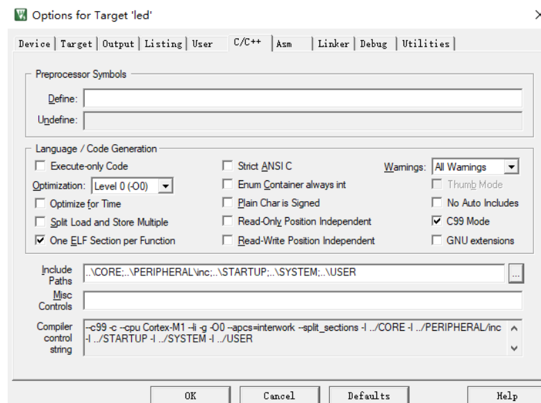
图 1-5 配置头文件路径
