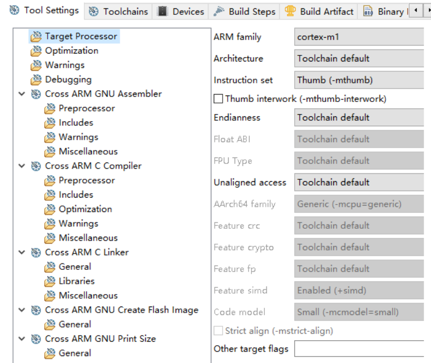
图 2-4 配置 Target Processor
