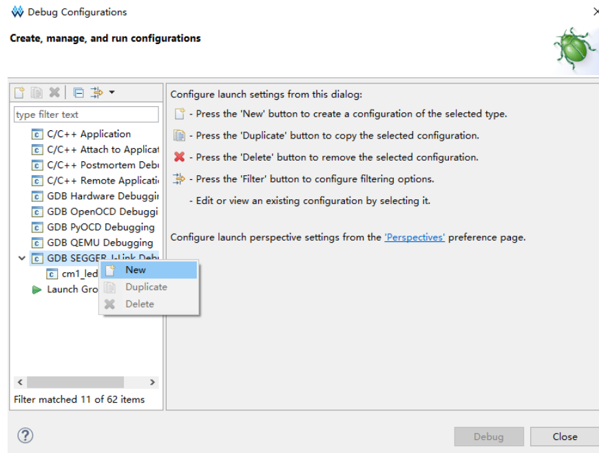
图 2-11 建立软件调试配置选项
