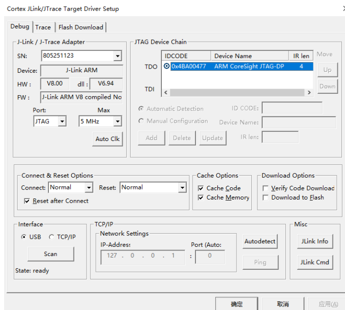
图 1-6 配置 JTAG 调试接口类型
