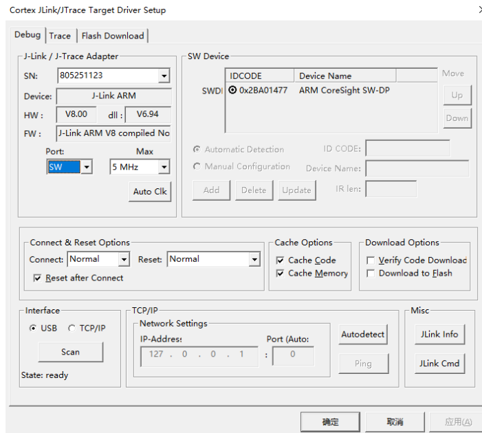
图 1-7 配置 SW 调试接口类型
