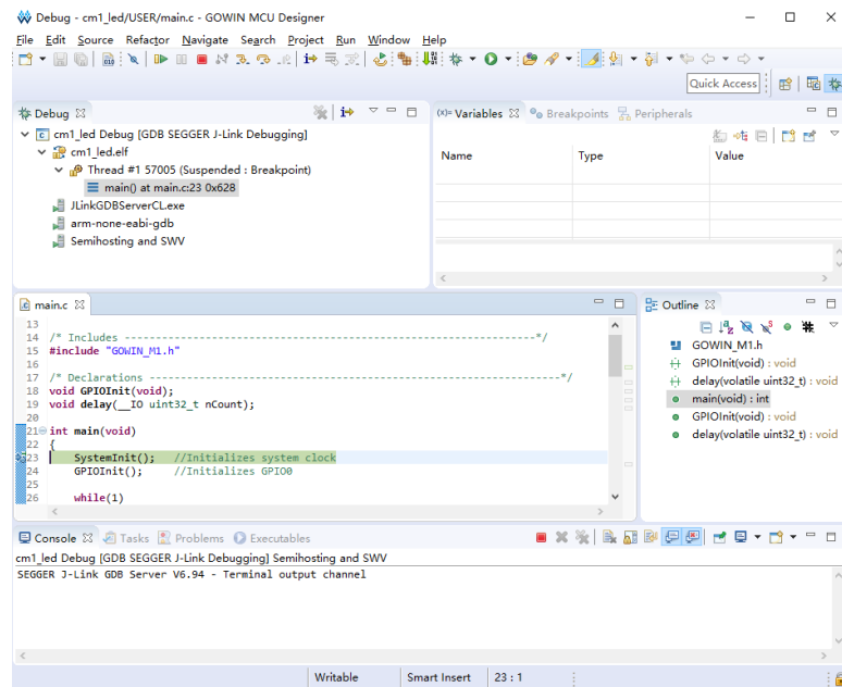
图 2-15 启动软件在线调试
