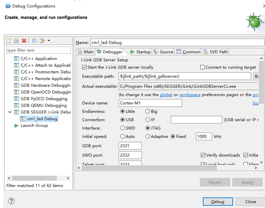
图 2-13 配置 Debugger 选项
