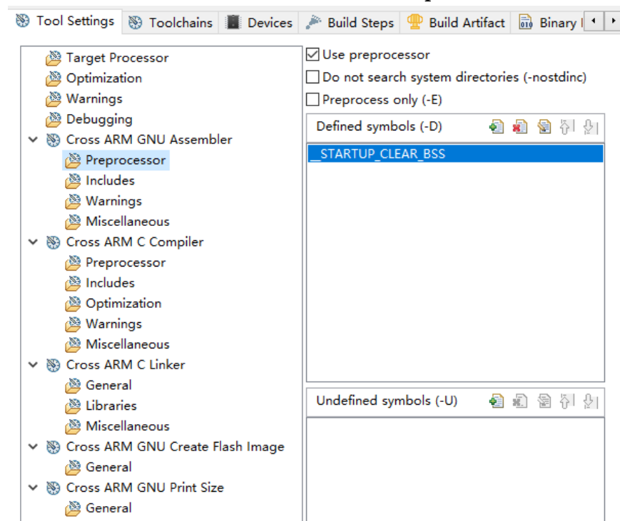
图 2-5 配置 Cross ARM GNU Assembler &gt; Preprocessor
