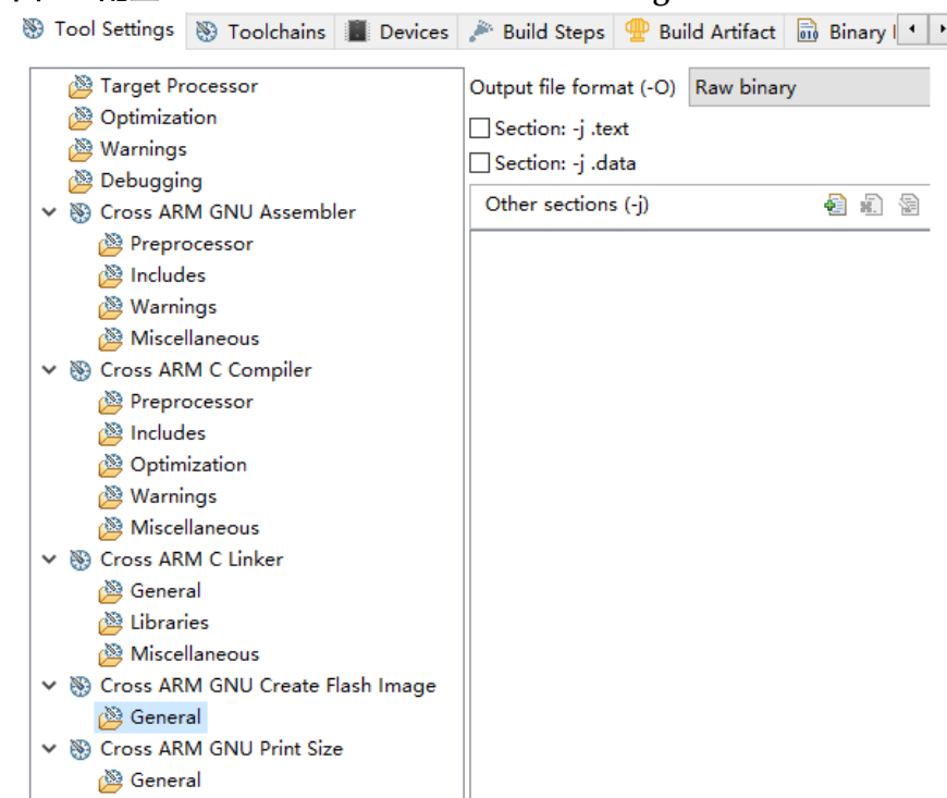
图 2-8 配置 Cross ARM GNU Create Flash Image
