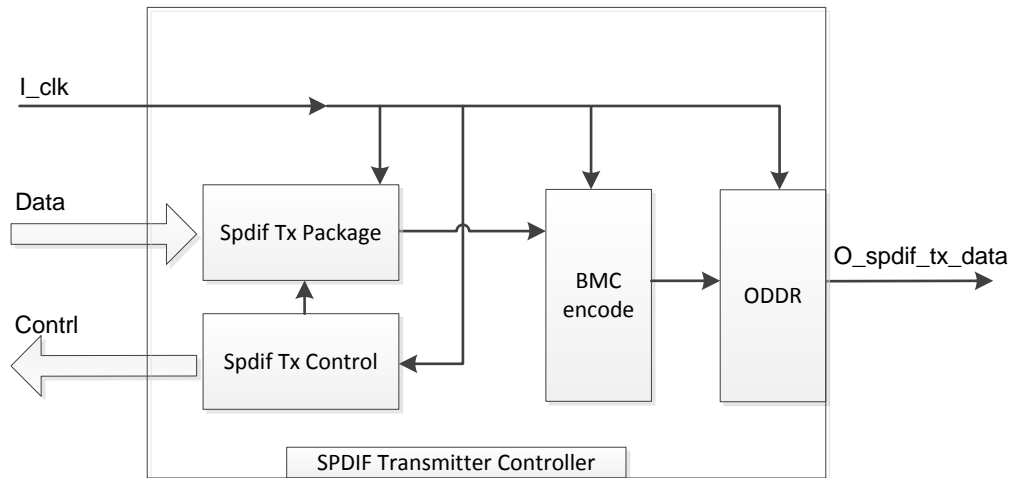
图 3-2 实现框图
