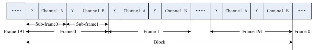
图 3-3 帧格式
