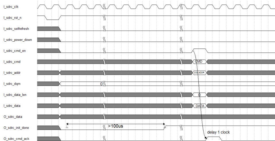
图 6-4 写操作时序（不带预充电）
