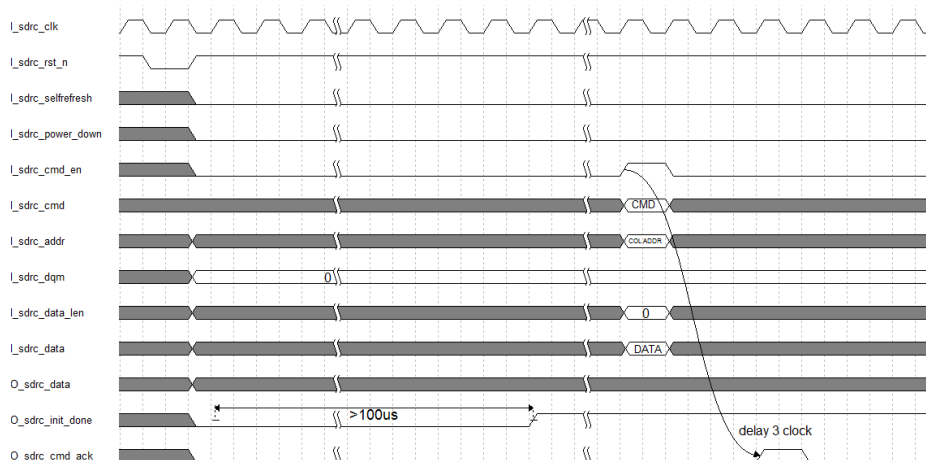
图 6-3 写操作时序（带预充电）
