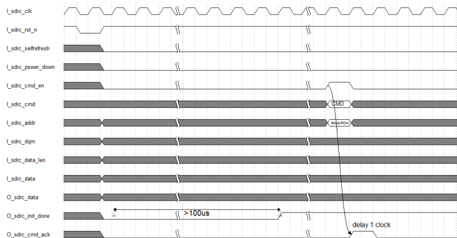
图 6-2 激活操作时序
