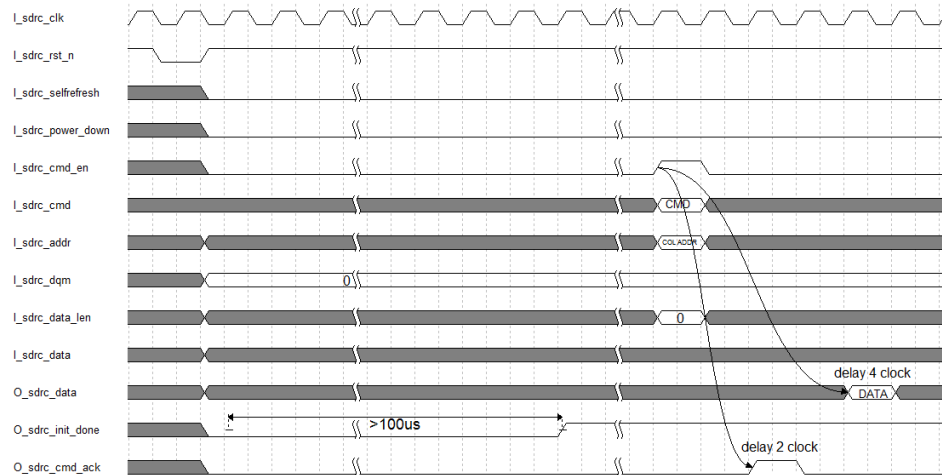
图 6-5 读操作时序（带预充电）
