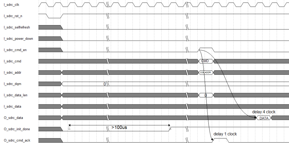
图 6-6 读操作时序（不带预充电）
