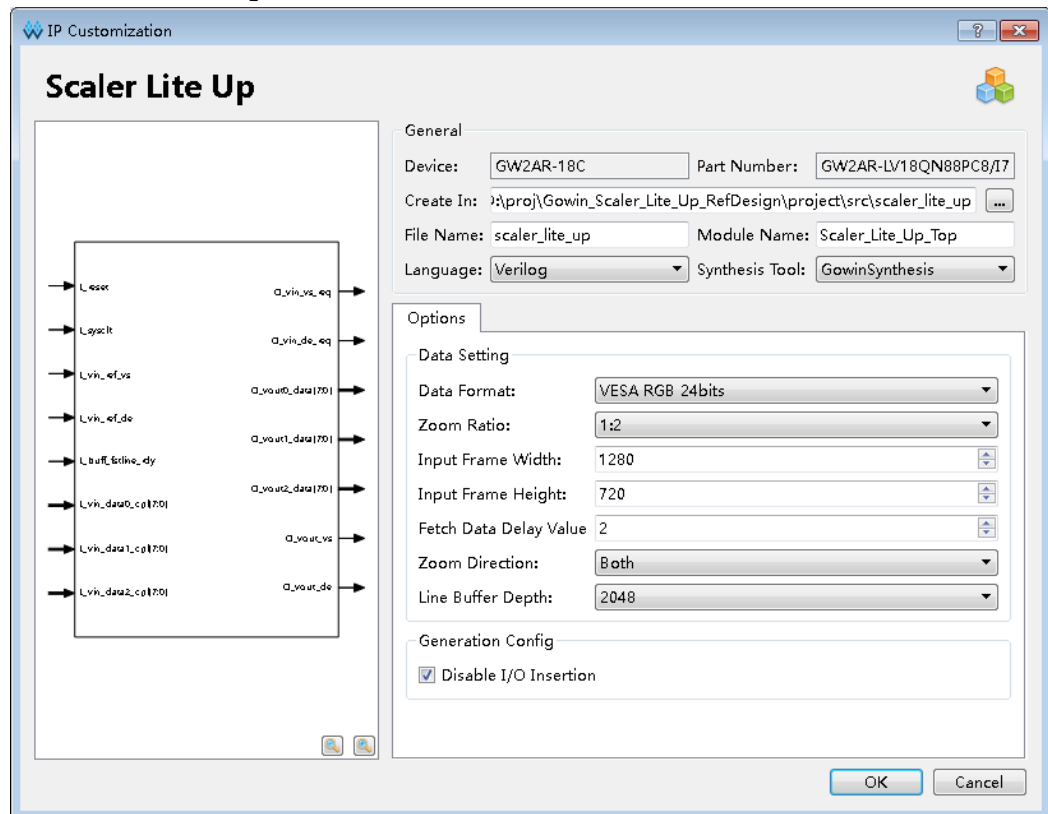
图 4-8 Scaler Lite Up IP 核接口示意图
