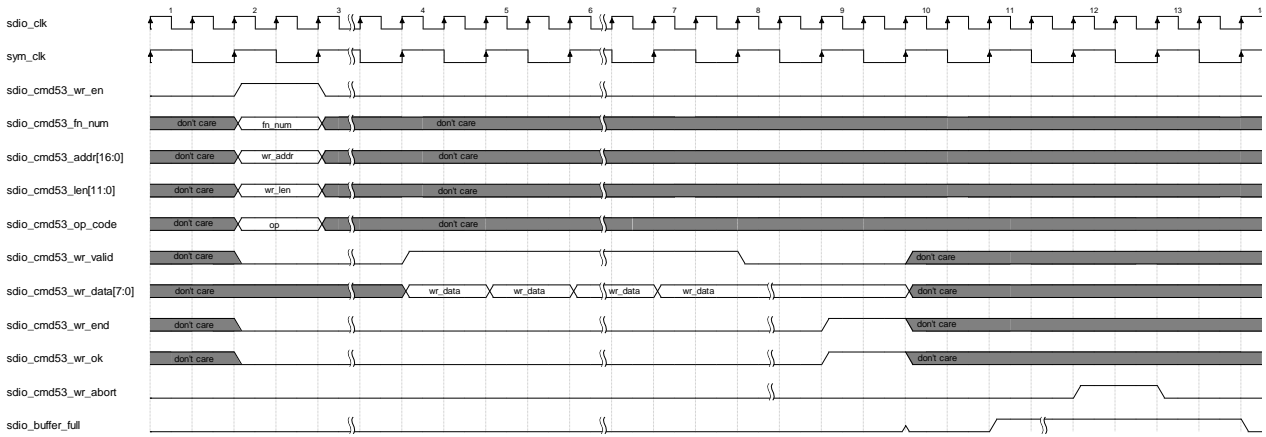
图 4-16 Write Good Abort Case2
