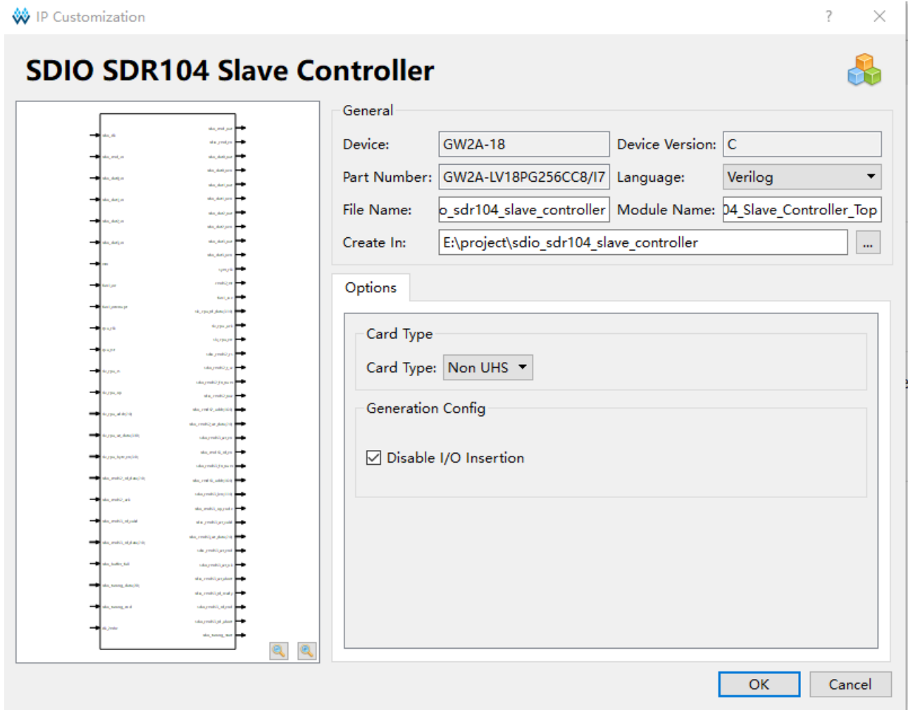
图 7-2 SDIO SDR104 Slave Controller IP 配置界面
