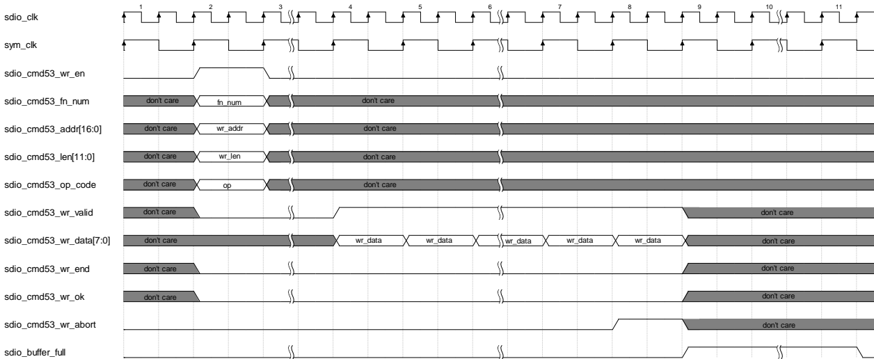
图 4-14 Write Bad Abort
