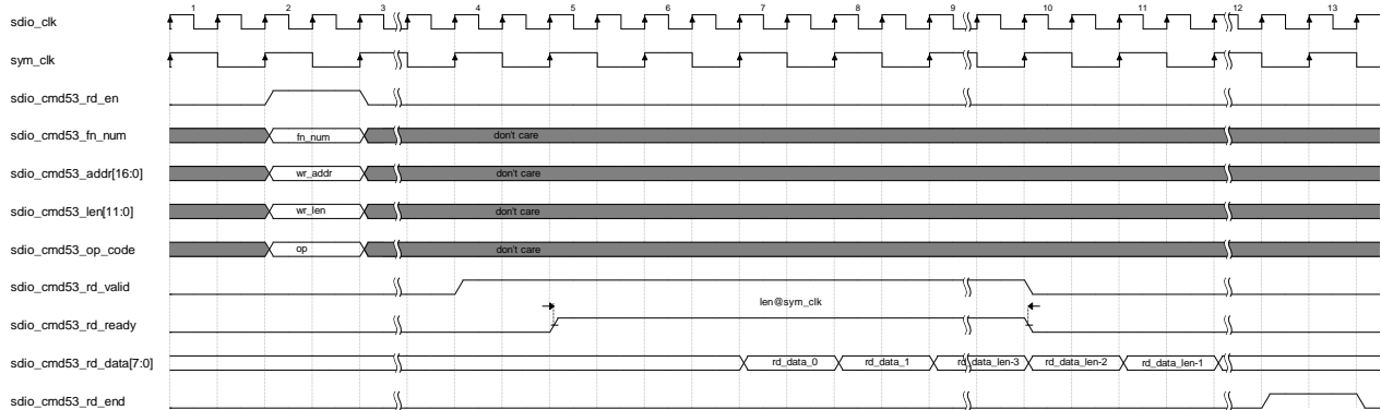
图 4-13 SDIO SDR104 CMD53 Interface 接口 4-bit 模式读操作
