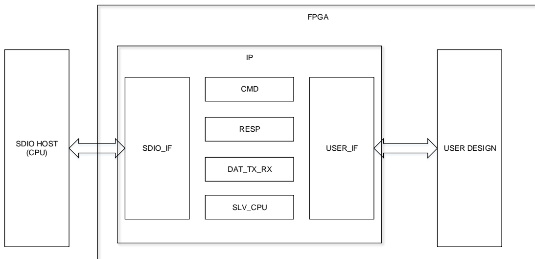
图 4-1 Gowin SDIO SDR104 Slave Controller IP 结构图
