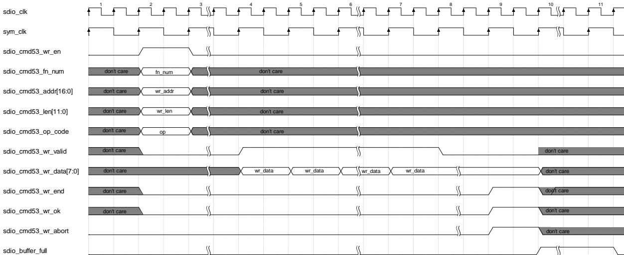
图 4-15 Write Good Abort Case1
