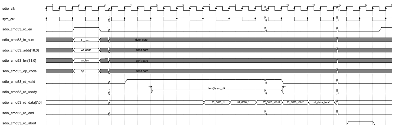
图 4-17 Read Bad Abort
