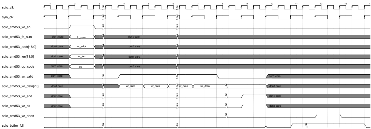
图 4-16 Write Good Abort Case2
