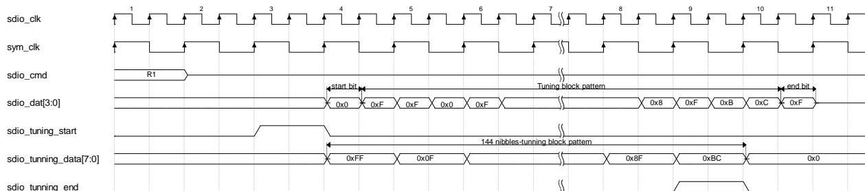
图 4-20 SDIO Tuning Interface 时序
