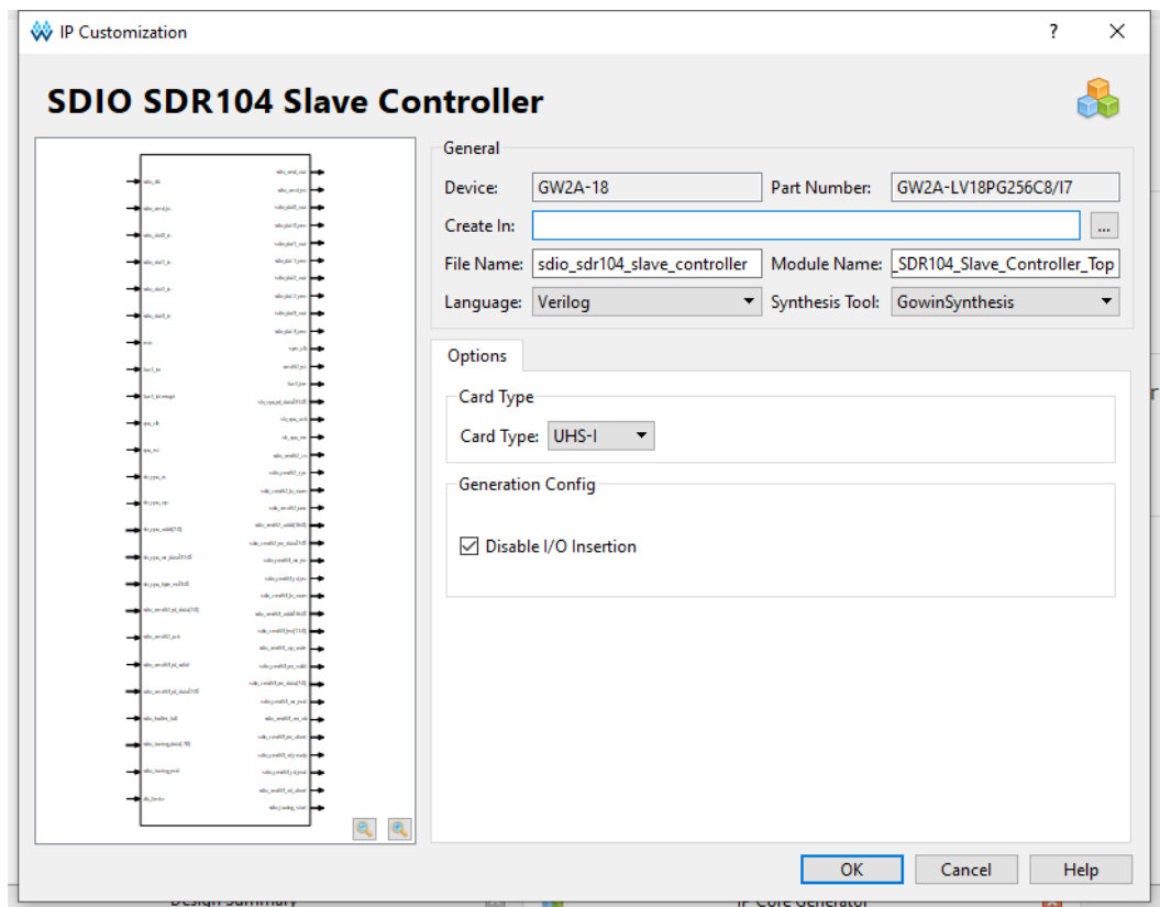
图 7-2 SDIO SDR104 Slave Controller IP 配置界面
