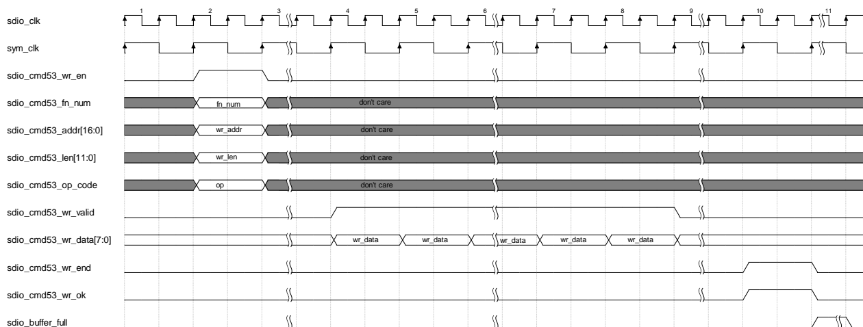
图 4-12 SDIO CMD53 Interface 接口 4-bit 模式写操作时序
