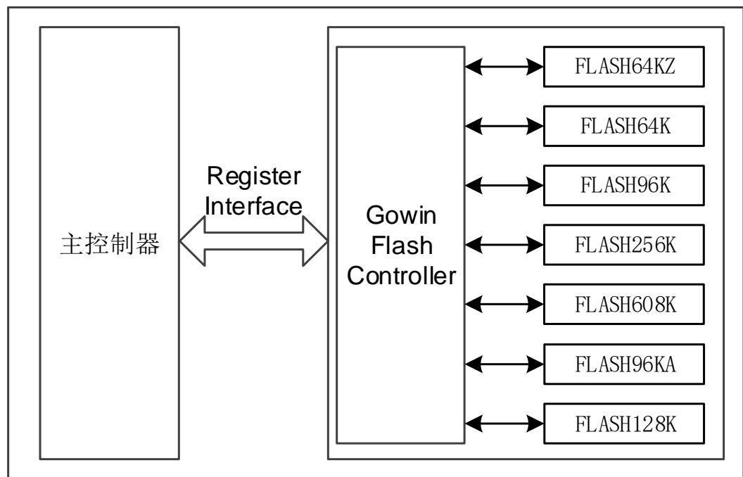
图 5-1 Register 接口
