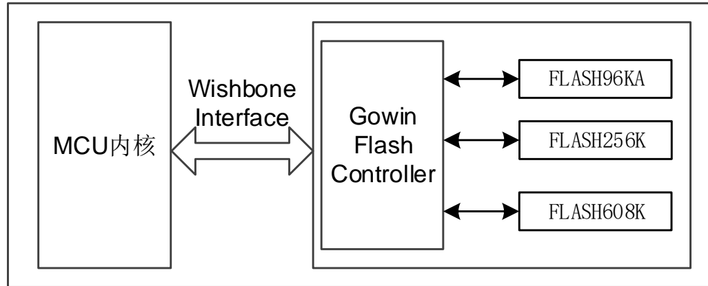
图 5-2 Wishbone 接口
