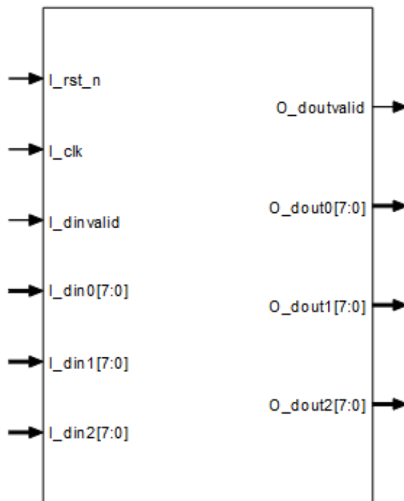
图 4-1 CSC IP 端口示意图
