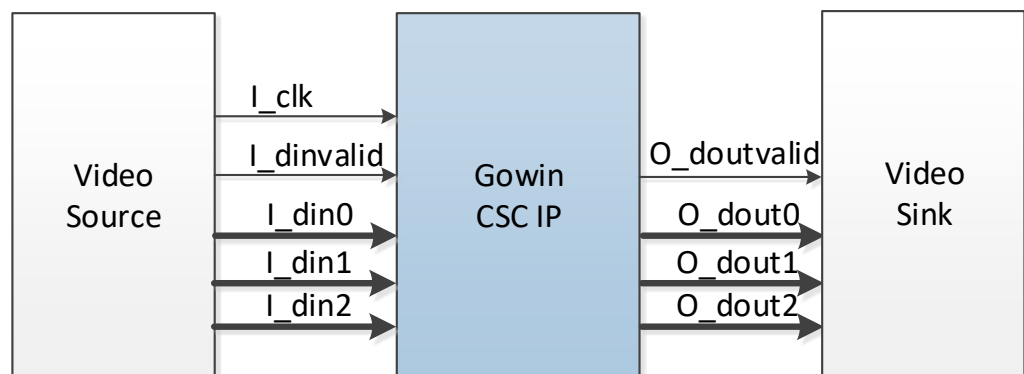
图 3-1 系统框图
