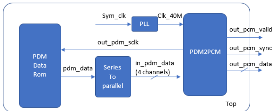
图 8-1 参考设计结构框图
