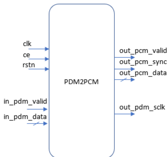
图 5-1 PDM2PCM IP 端口图
