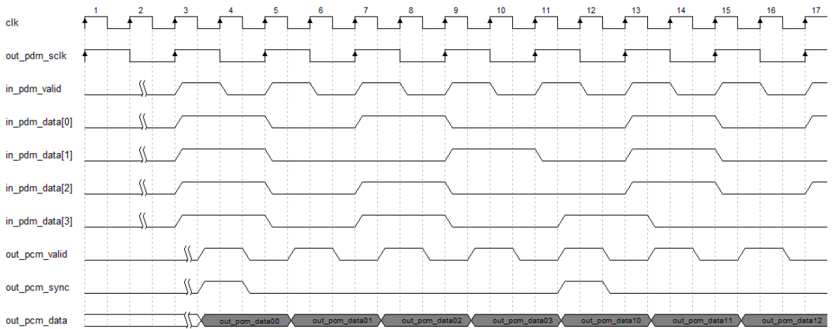
图 6-1 PDM2PCM(4 通道)状态时序图
