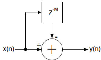
图 2-3 Comb Filter
