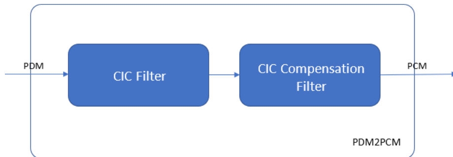
图 4-1 PDM2PCM 实现框图
