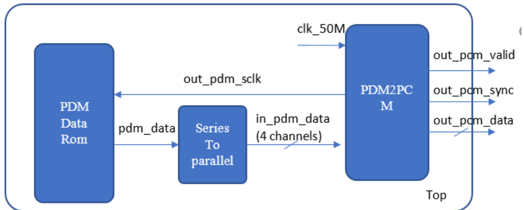
图 8-1 参考设计结构框图
