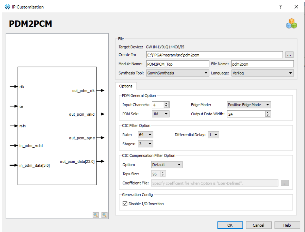
图 7-2 IP PDM2PCM 配置界面
