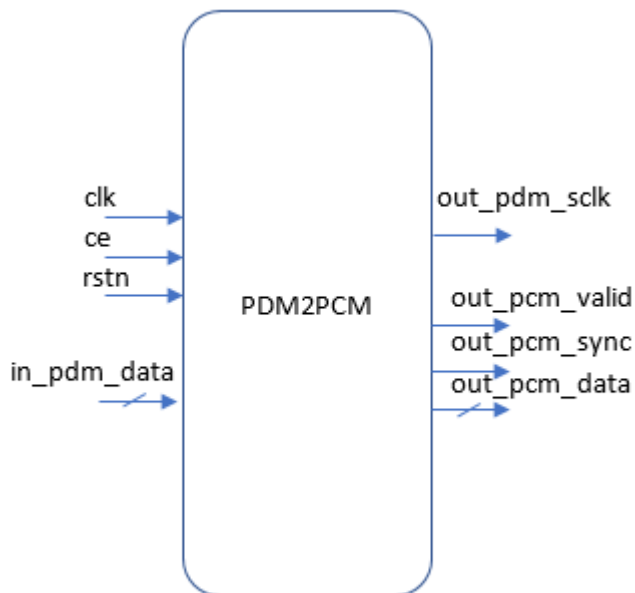
图 5-1 PDM2PCM IP 端口图
