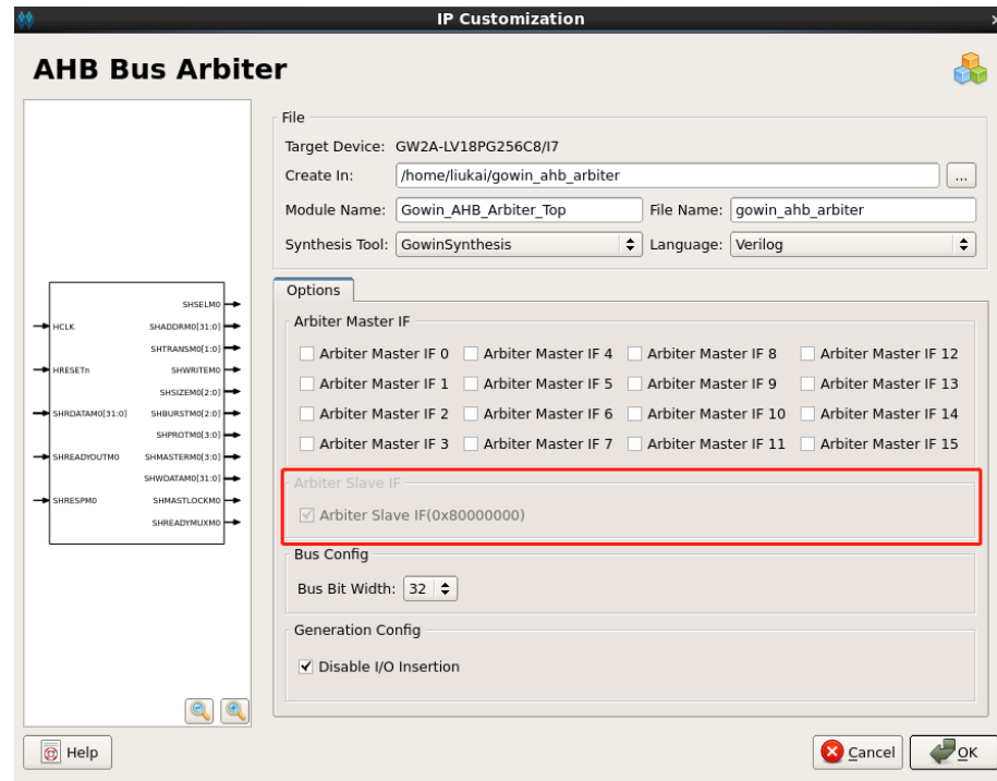
图 6-3 Arbiter Slave IF 配置
