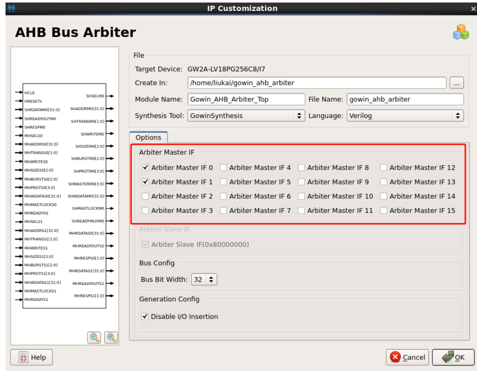
图 6-2 Arbiter Master IF 配置
