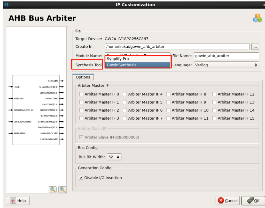
图 6-5 综合工具配置
