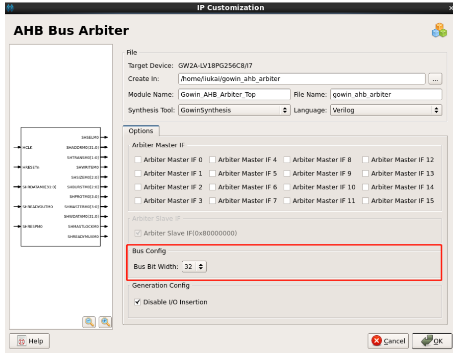
图 6-4 Bus Bit Width 配置
