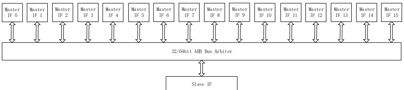
图 3-1 AHB 总线仲裁器模型
