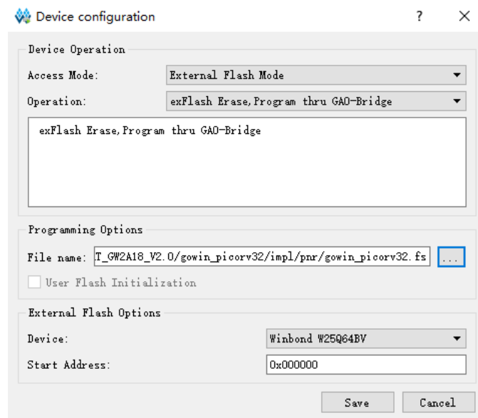
图 3-26 GW2A 系列 Configure Device
