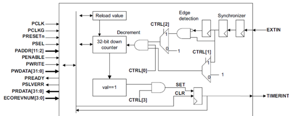
图 5-1 Timer
