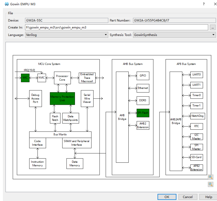
图 3-6 系统架构图
