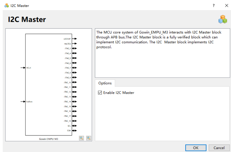
图 3-20 I2C Master 配置
