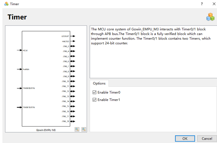
图 3-17 Timer 配置
