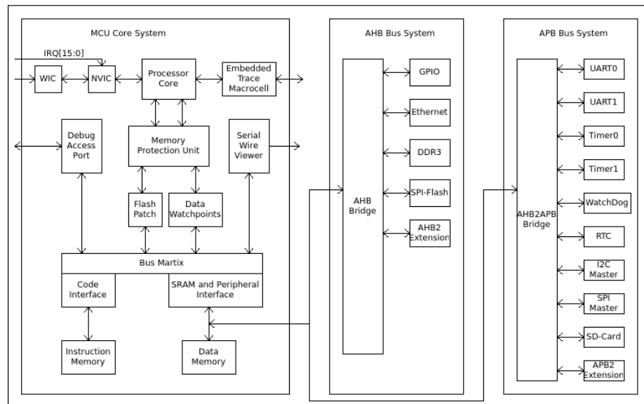
图 1-1 系统架构
