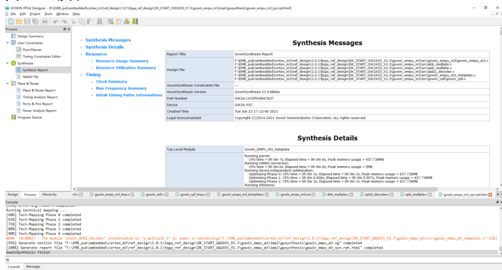
图 3-25 综合
