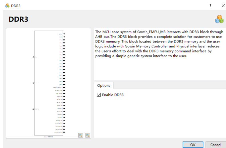
图 3-13 DDR3 配置
