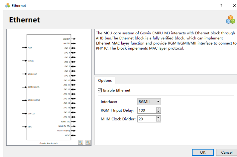
图 3-12 Ethernet 配置
