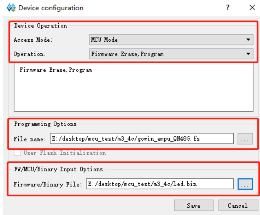
图 1-8 器件 GW1NS-4C 或 GW1NSR-4C 下载选项配置
