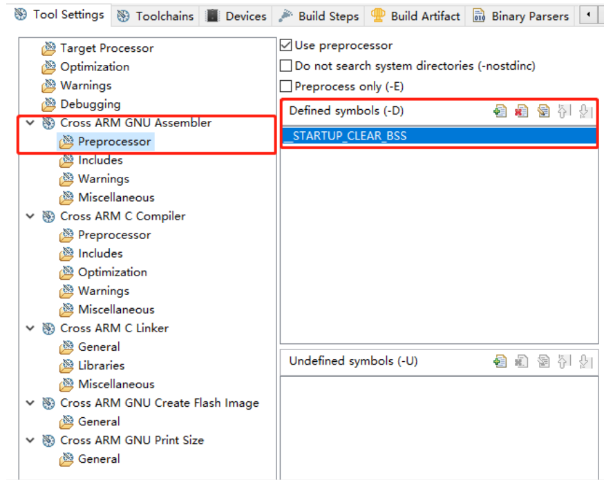
图 2-5 配置 Cross ARM GNU Assembler > Preprocessor 选项
