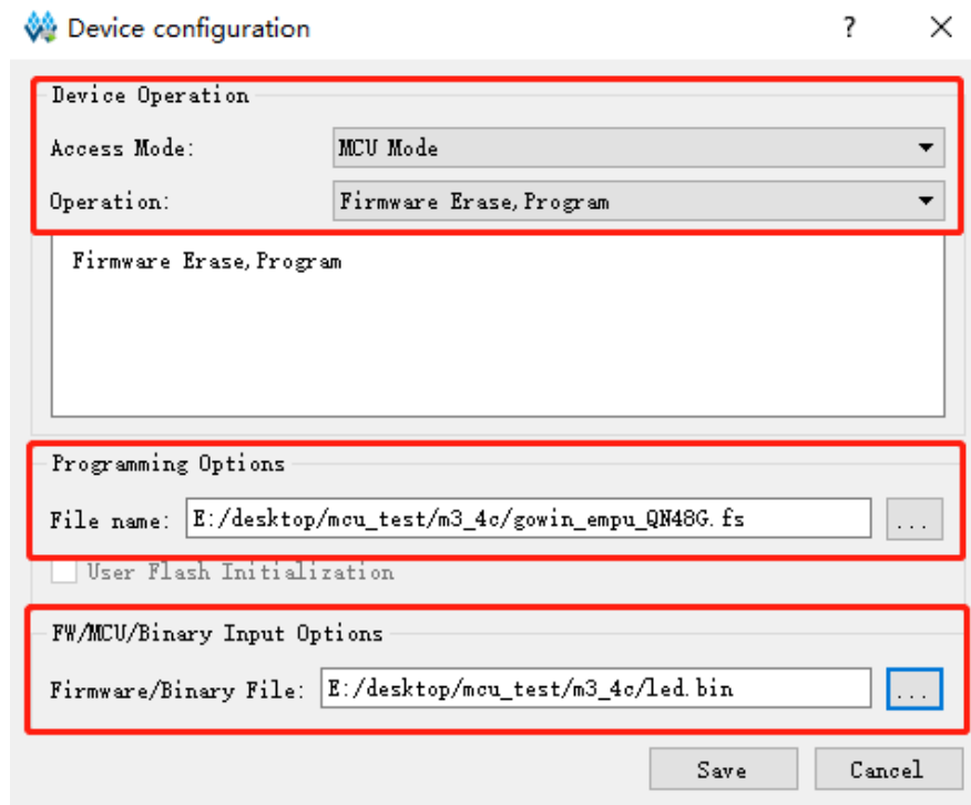
图 2-12 器件 GW1NS-4C 或 GW1NSR-4C 下载选项配置
