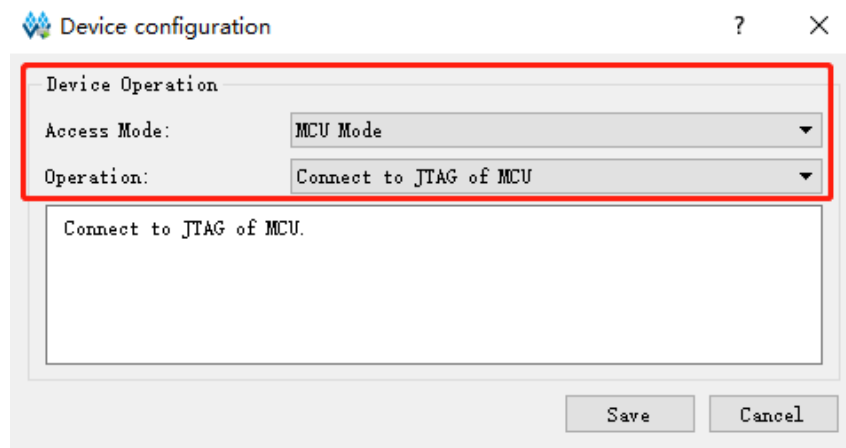
图 1-10 器件 GW1NS-4C 或 GW1NSR-4C MCU JTAG 模式切换配置
