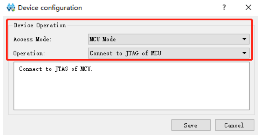
图 2-18 器件 GW1NS-4C 或 GW1NSR-4C MCU JTAG 模式切换配置
