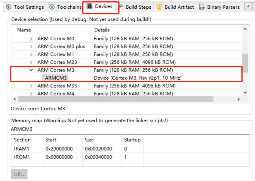
图 2-9 配置 Devices 选项
