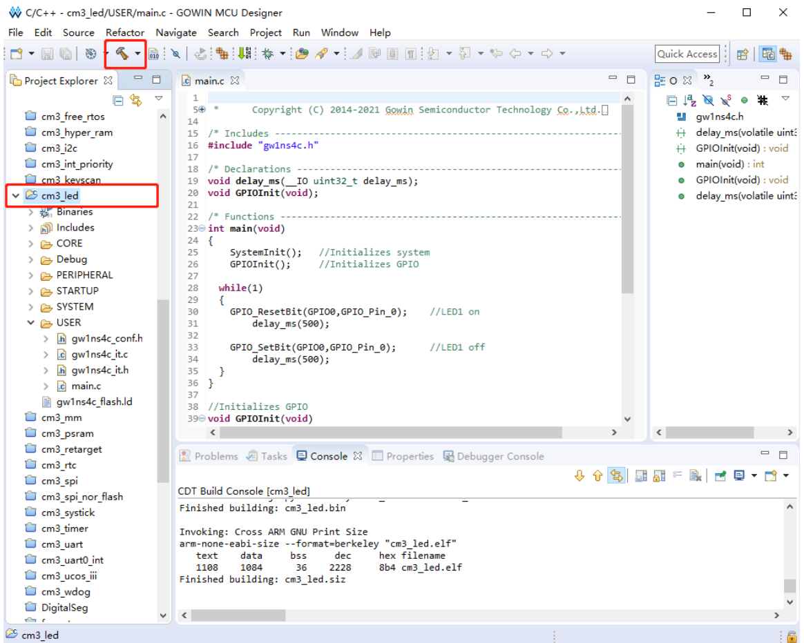
图 3-2 编译
