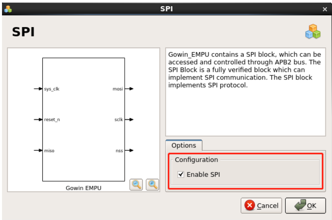
图 3-14 SPI 配置
