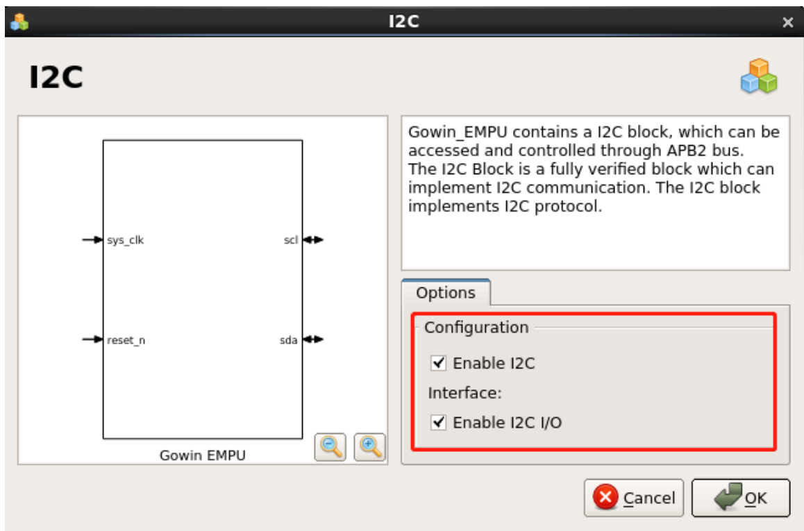
图 3-13 I2C 配置
