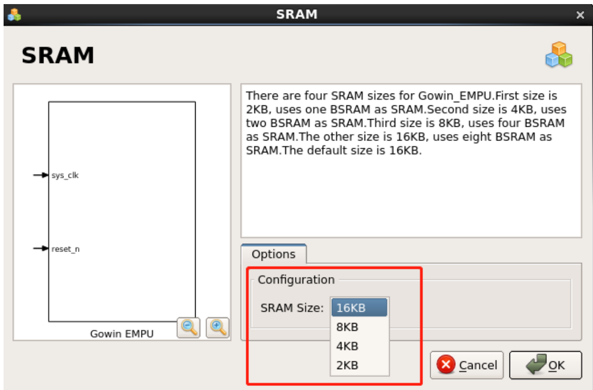
图 3-12 SRAM 配置
