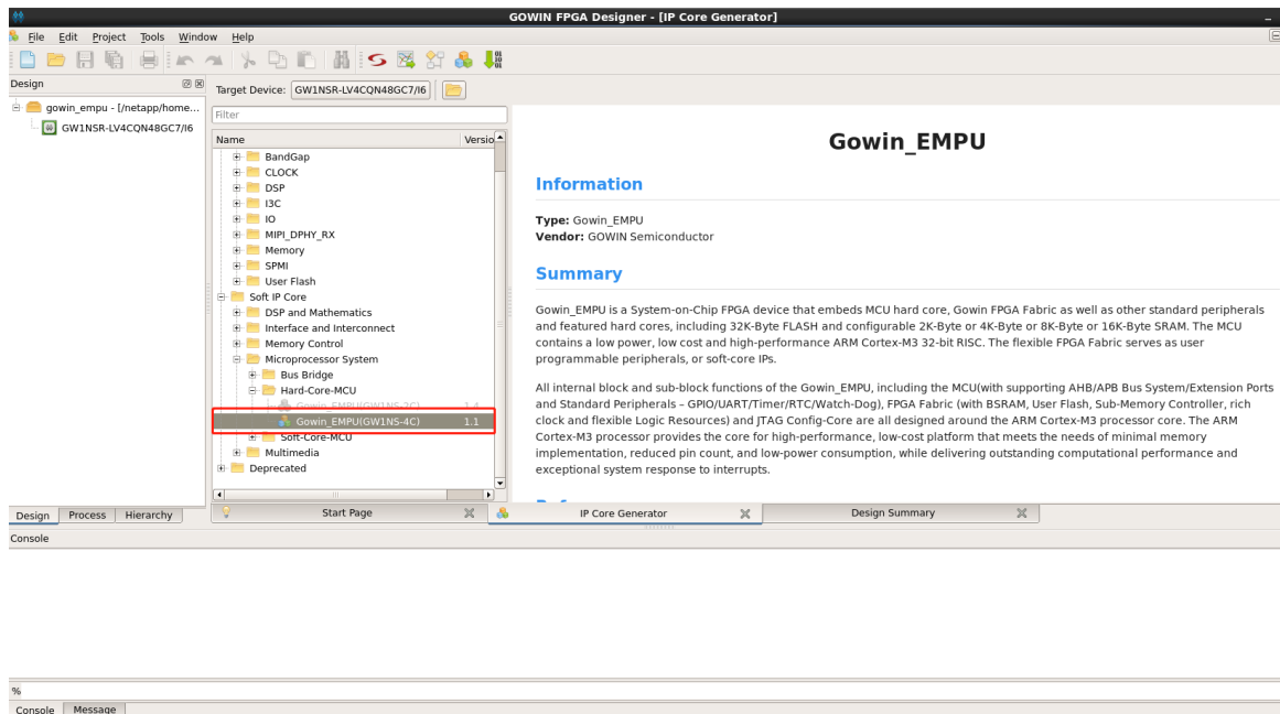
图 3-5 选择 Gowin_EMPU(GW1NS-4C)
