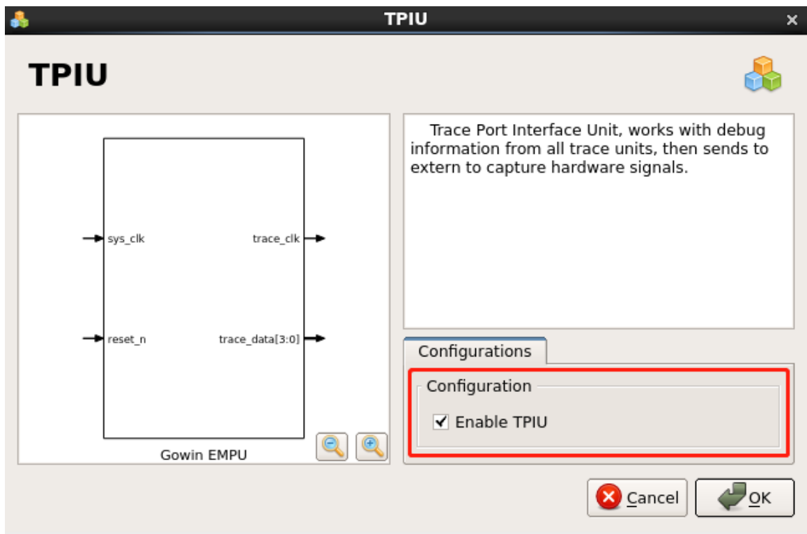
图 3-7 TPIU 配置
