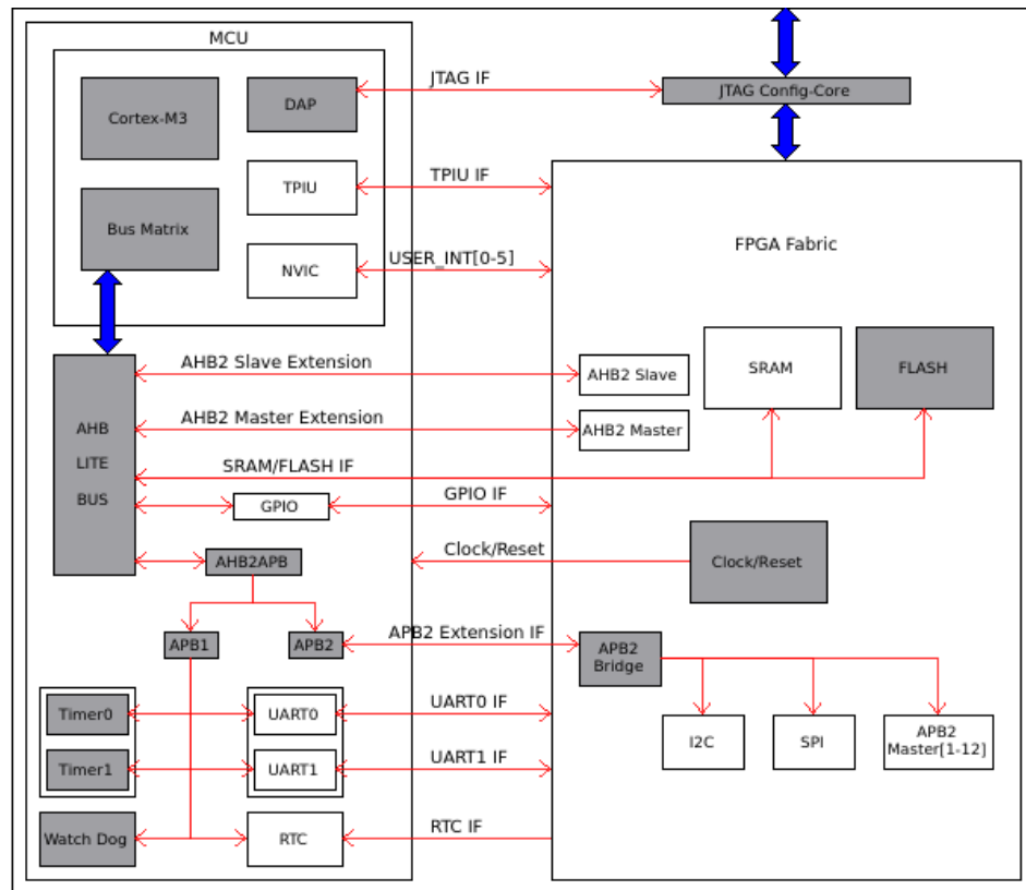
图 1-1 系统架构
