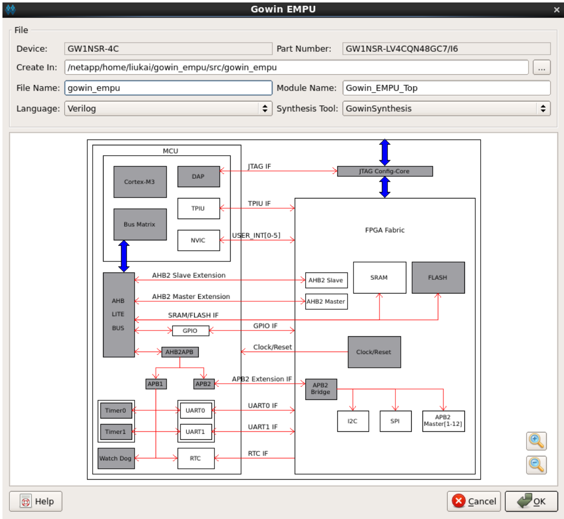
图 3-6 系统结构图
