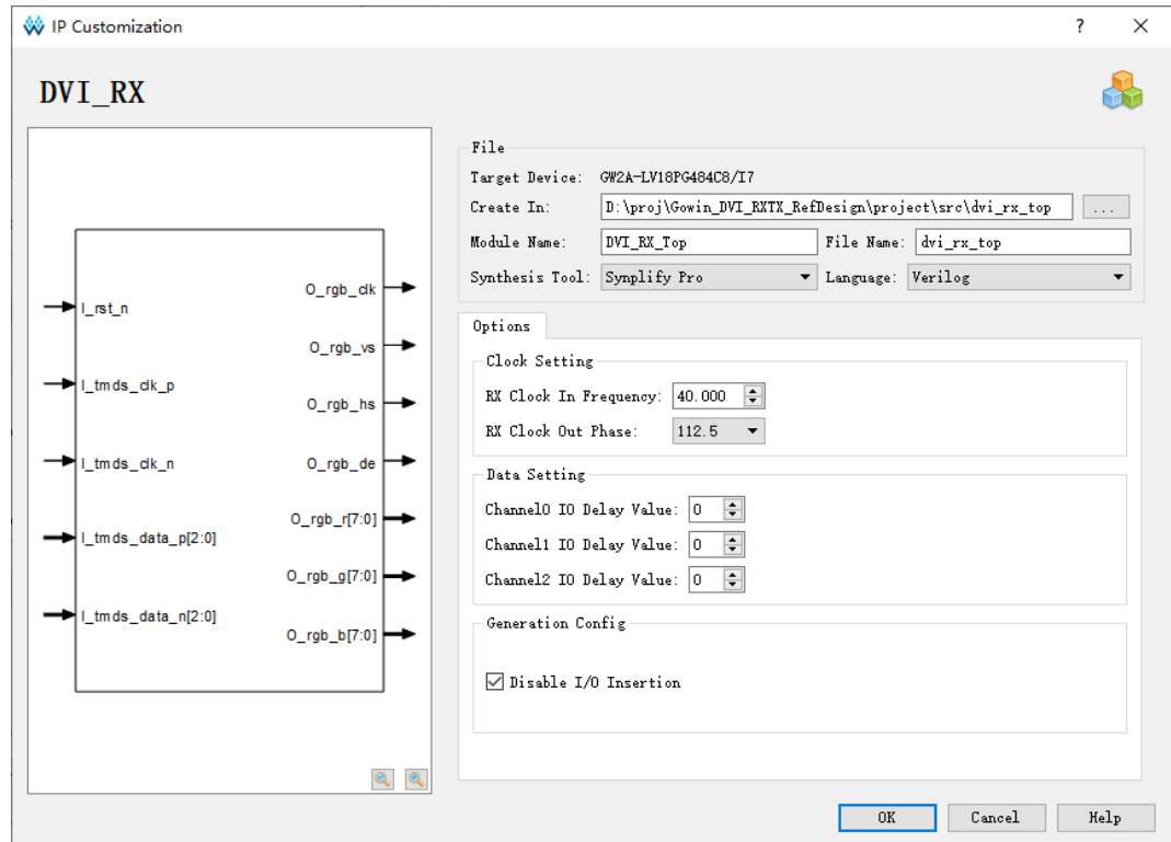
图 4-9 DVI RX IP 核接口示意图
