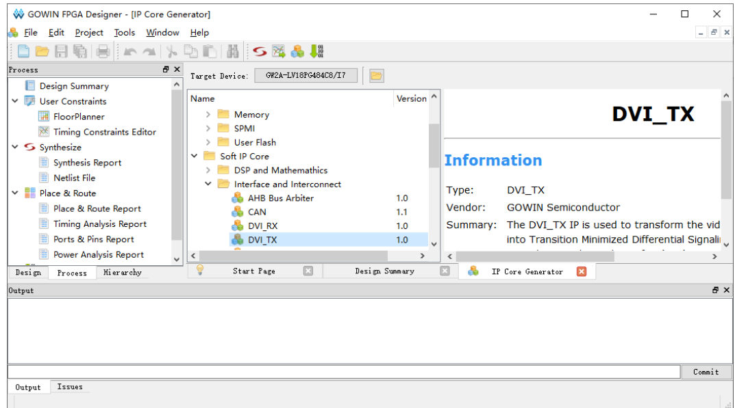
图 4-2 打开 DVI TX IP 核
