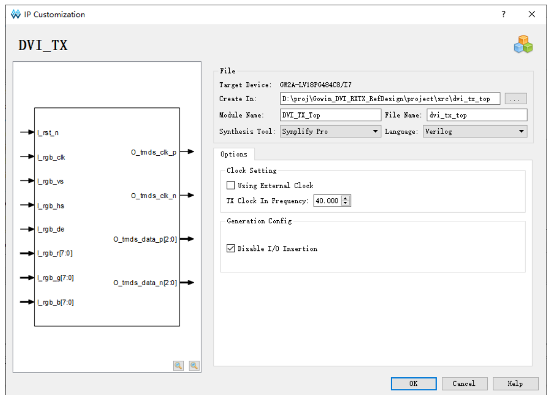
图 4-3 DVI TX IP 核接口示意图
