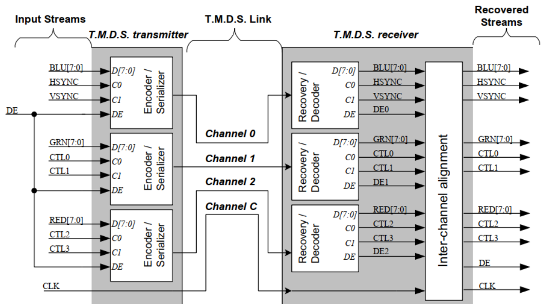
图 3-2 实现框图
