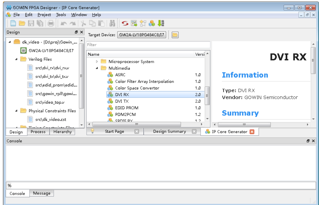
图 4-8 打开 DVI RX IP 核
