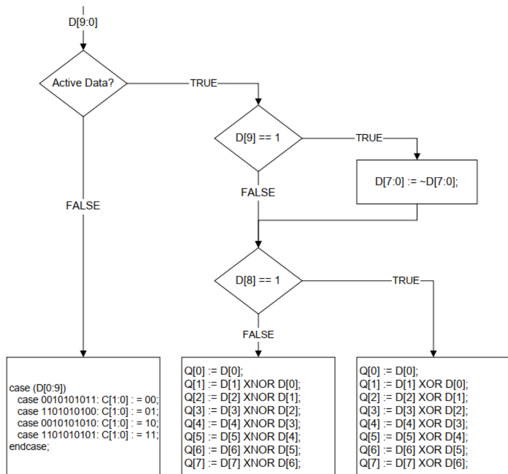
图 3-4 TMDS 解码算法流程图
