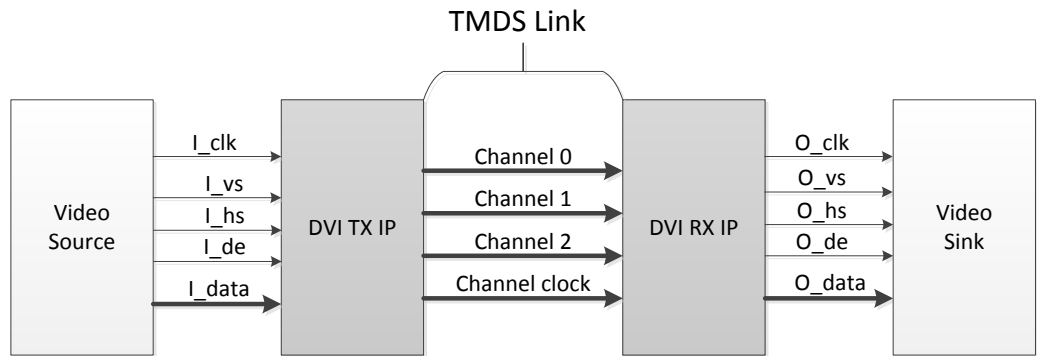
图 3-1 系统框图
