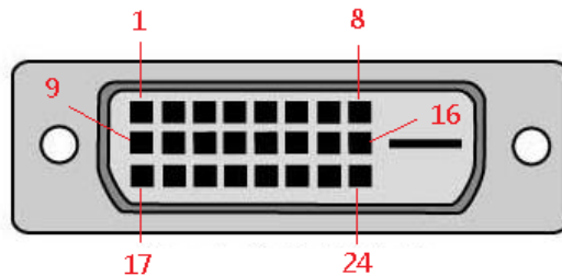
DVI-D 连接器
