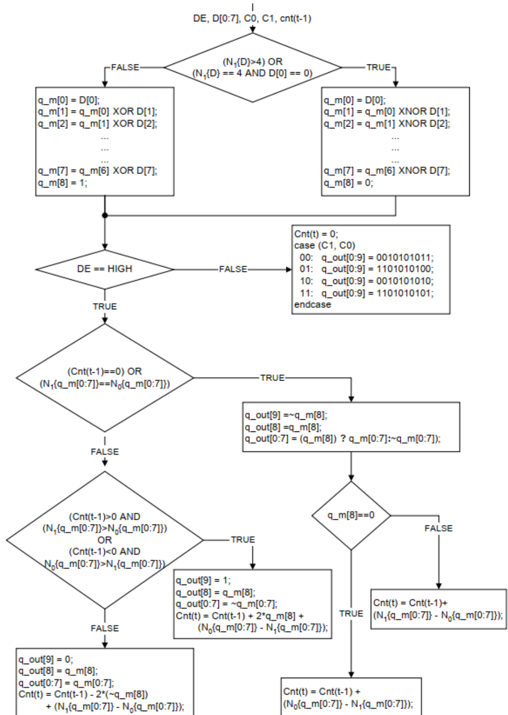
图 3-3 TMDS 编码算法流程图
