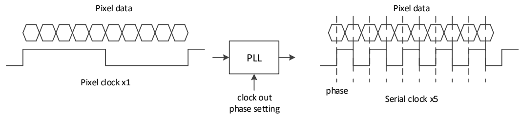
图 3-9 DVI RX 串行数据采样示意图
