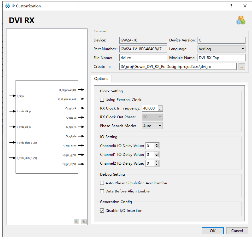
图 4-8 DVI RX IP 核接口示意图
