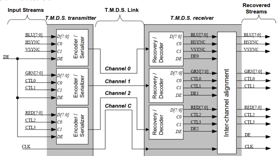
图 3-2 实现框图
