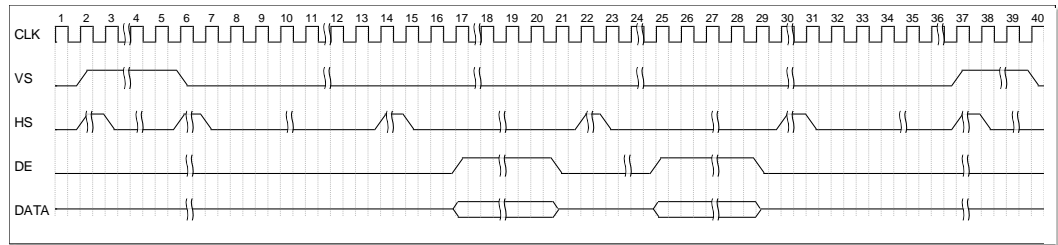
图 3-7 DVI 视频接口时序示意图
