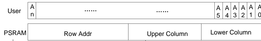
图 4-5 Row-Column 顺序的寻址方案
