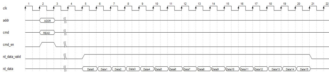
图 4-13 突发长度为 64 时读数据时序图
