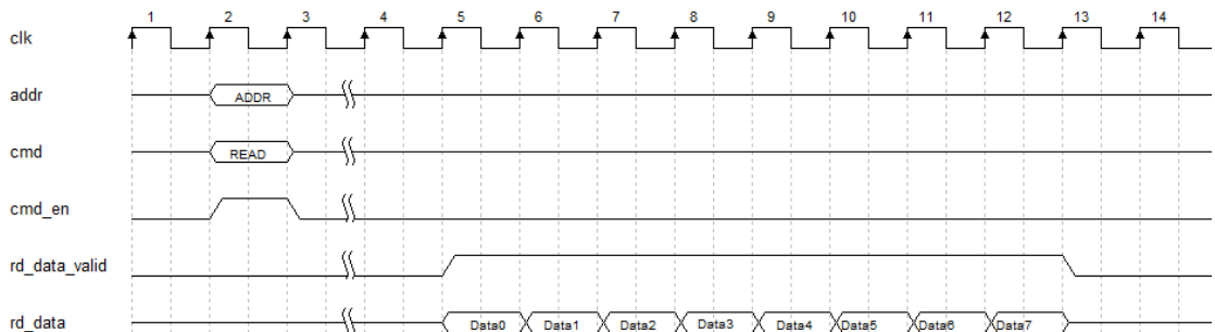
图 4-12 突发长度为 32 时读数据时序图
