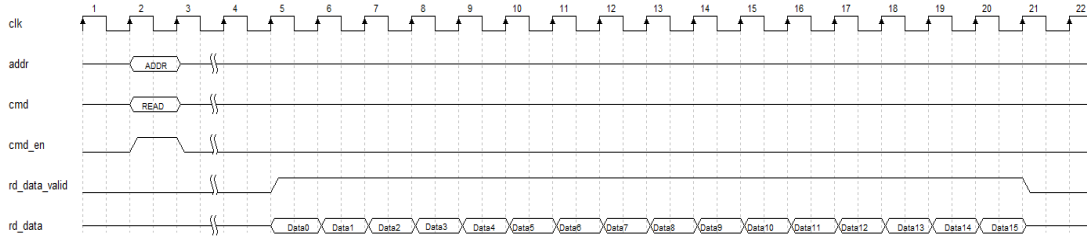
图 4-13 突发长度为 64 时读数据时序图
