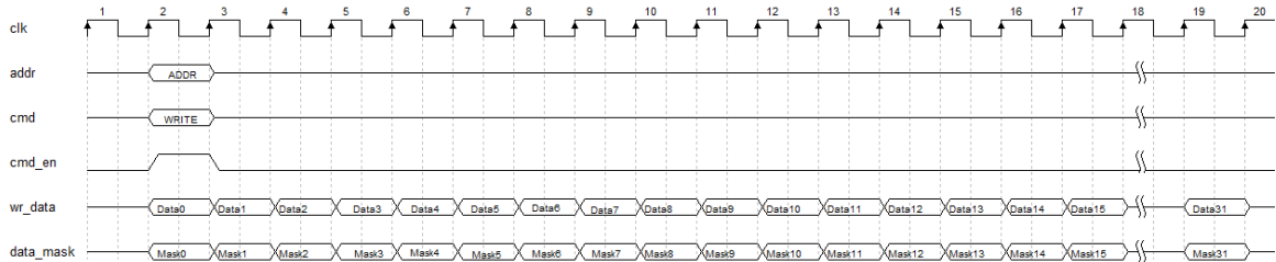
图 4-10 突发长度为 128 时写数据时序图
