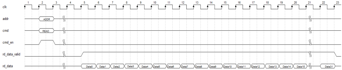
图 4-14 突发长度为 128 时读数据时序图
