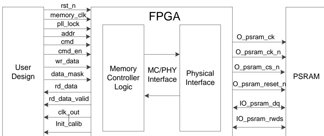
图 4-1 Gowin PSRAM Memory Interface HS IP 结构图
