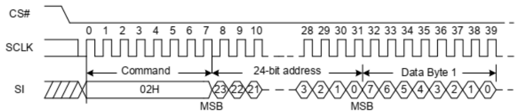
图 3-17 SPI Flash 写接口时序图
