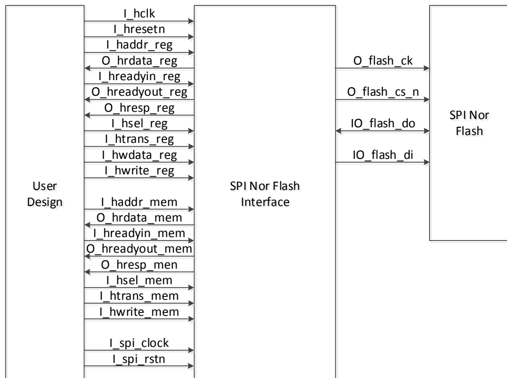
图 3-1 系统框图
