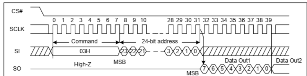
图 3-7 Read Data Bytes 时序图
