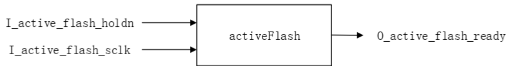
图 3-20 activeFlash 端口示意图
