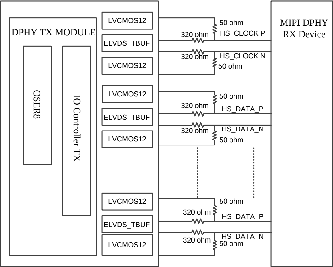
图 4-2 HS 模式和 LP 模式的接口实现，HS 采用 ELVDS
