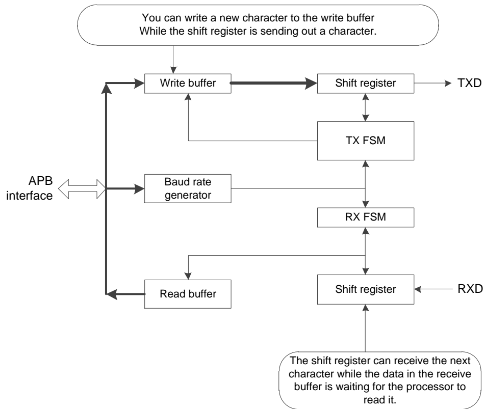
图 13-1 UART Buffering
