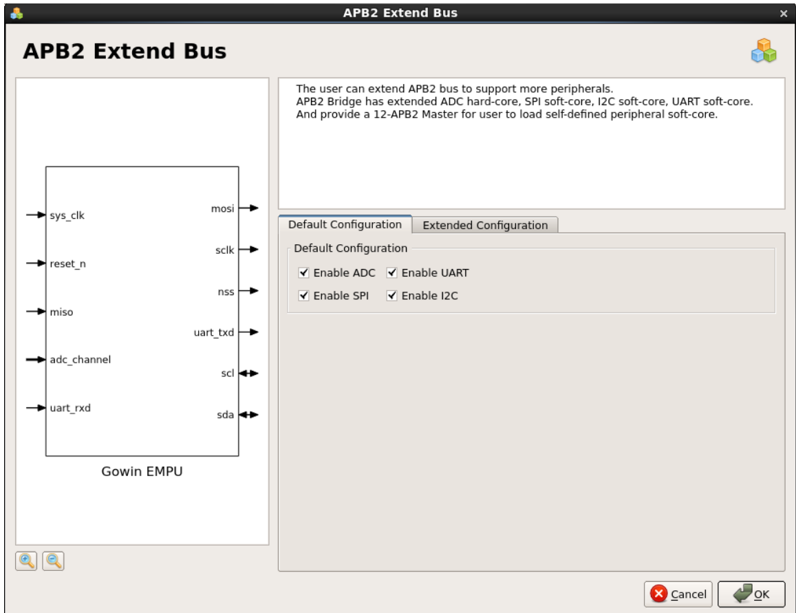
图 3-14 APB2 Extend Bus 默认配置
