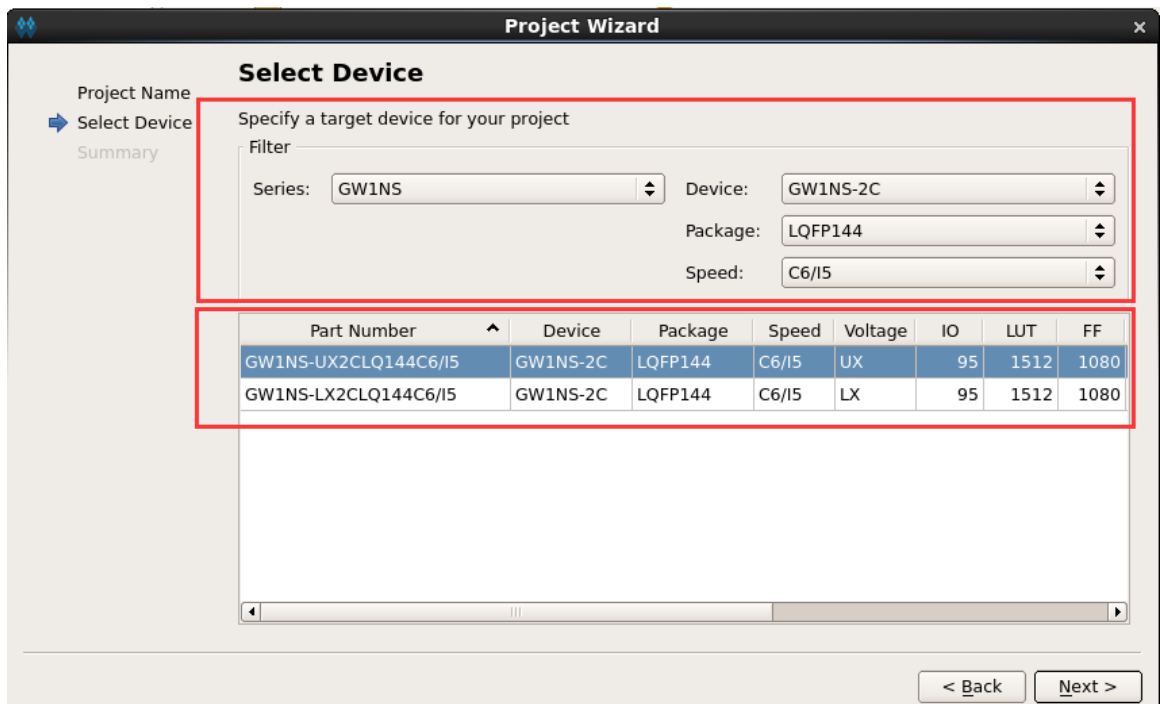
图 3-3 选择器件
