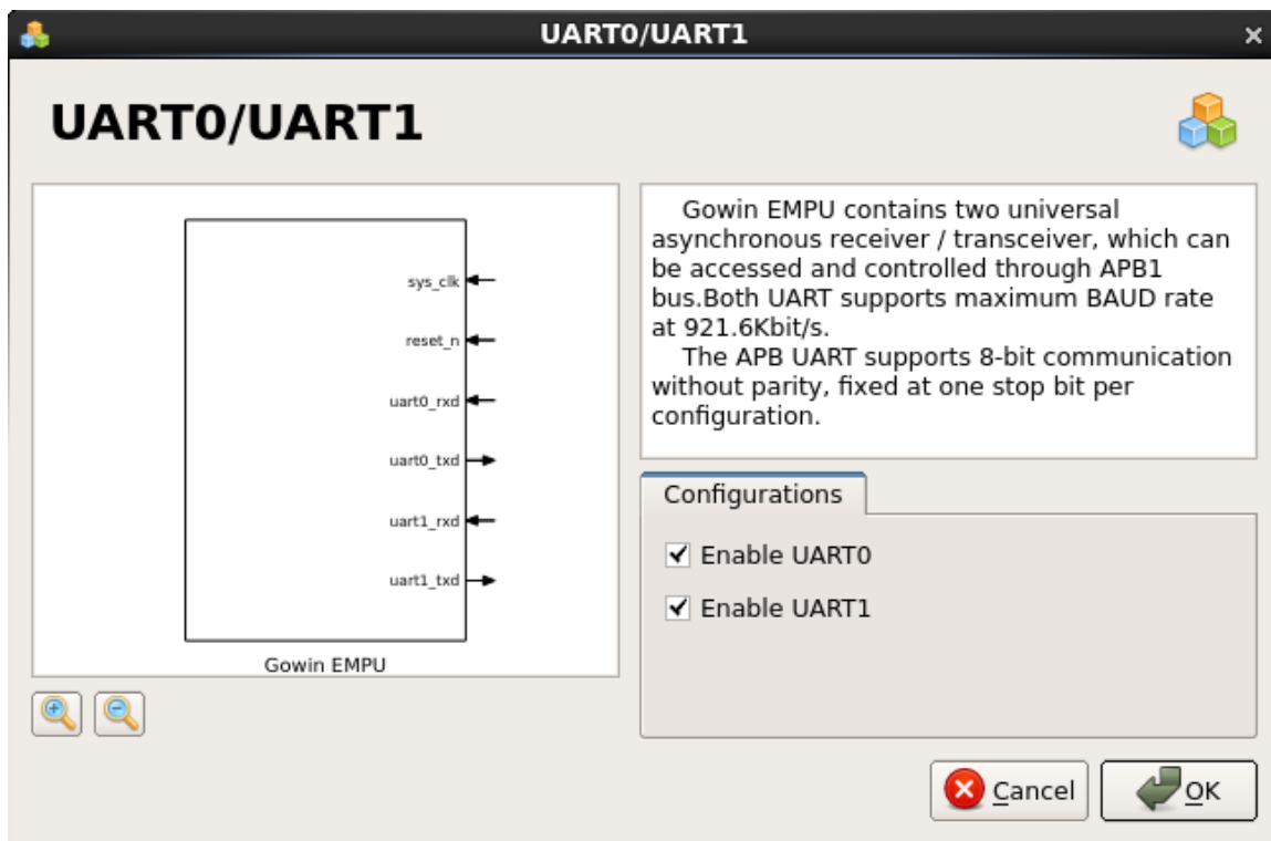
图 3-10 选择 UART
