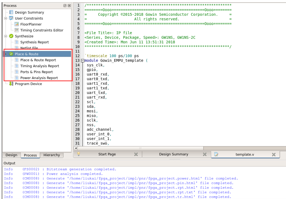
图 3-17 布局布线
