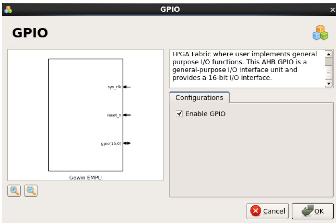
图 3-9 选择 GPIO
