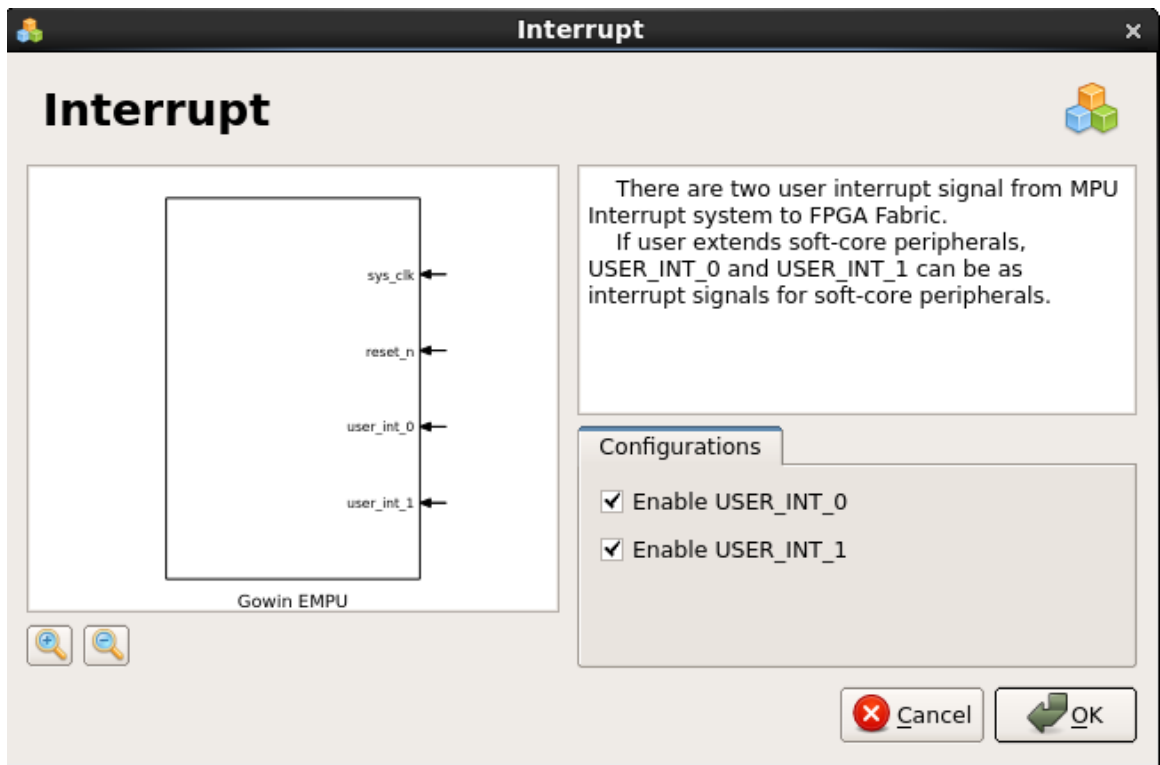
图 3-8 选择 Interrupt
