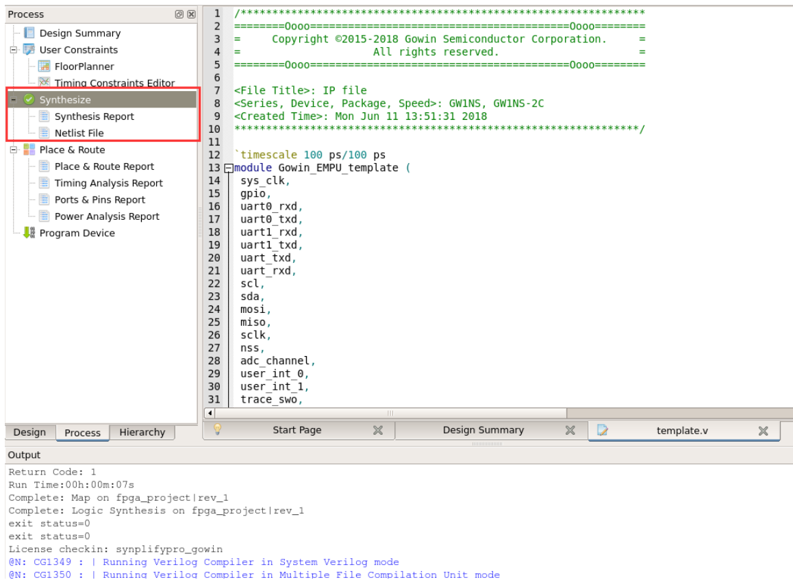
图 3-16 综合
