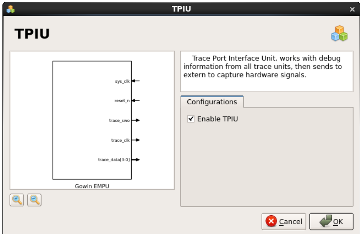
图 3-7 选择 TPIU
