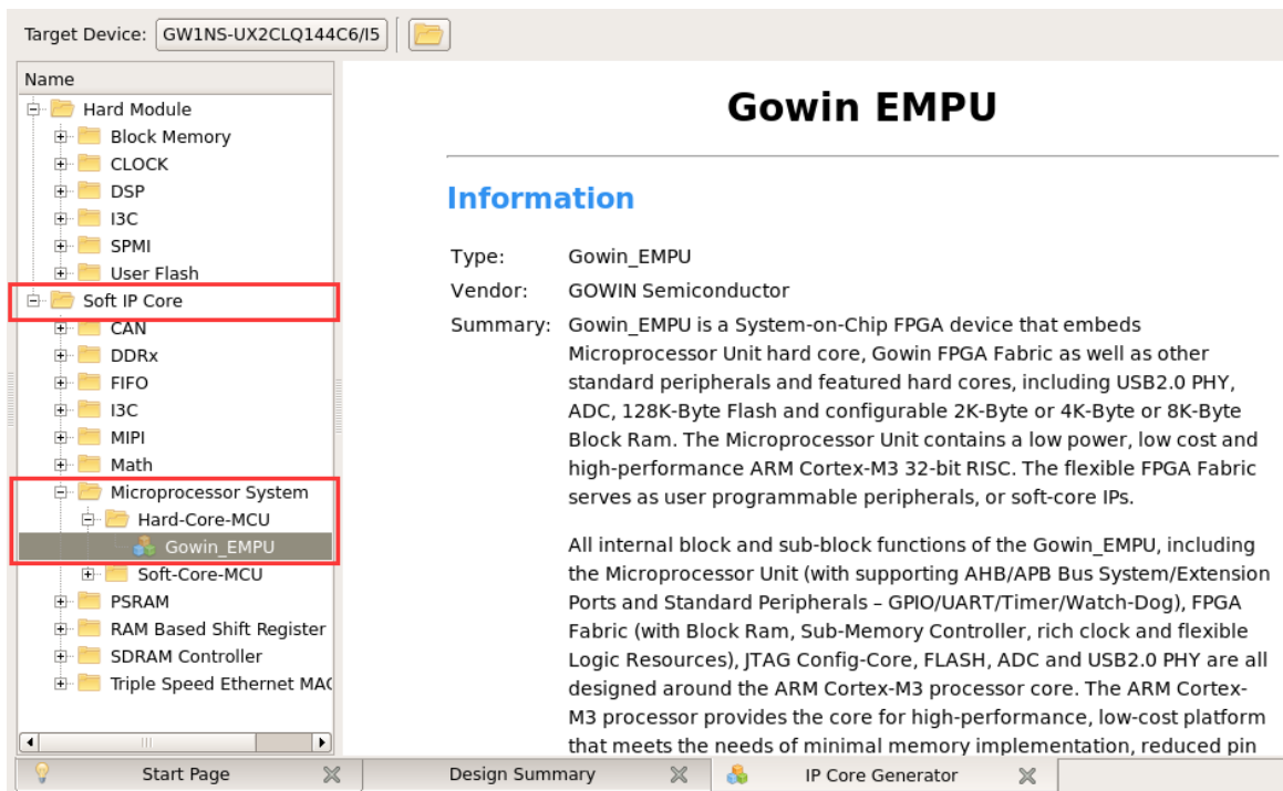
图 3-5 选择 Gowin_EMPU
