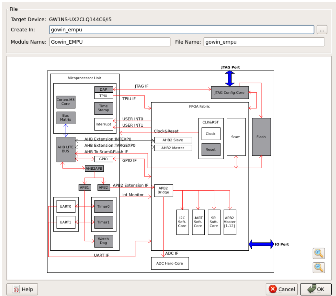
图 3-6 Gowin_EMPU
