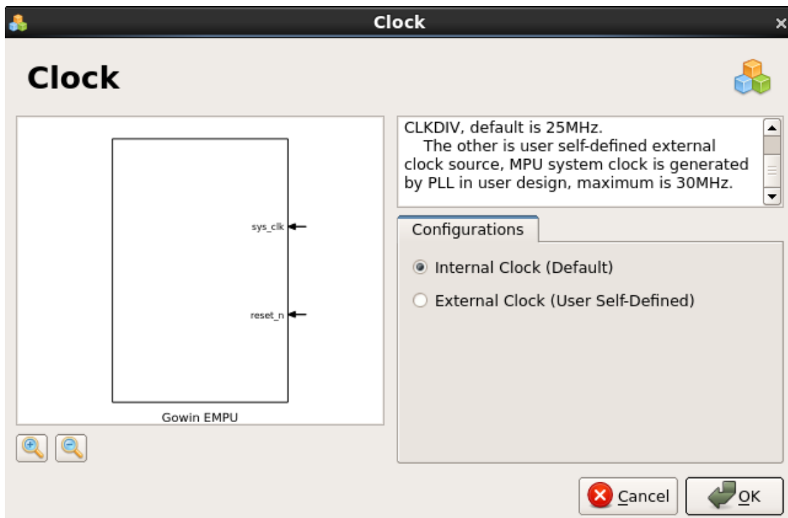
图 3-12 配置时钟
