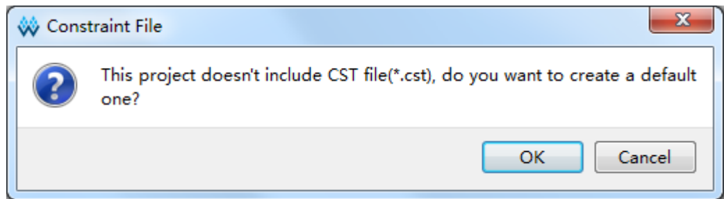
图 5-36 创建约束文件 Warning 提示
