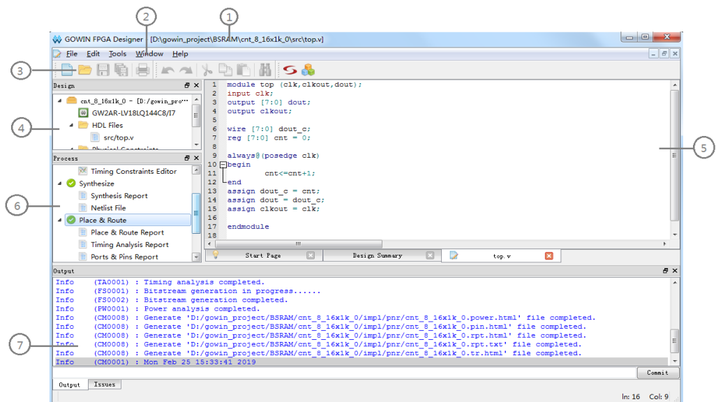
图 4-1 软件用户界面
