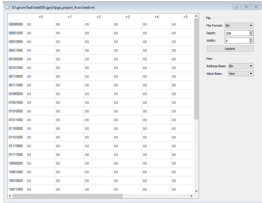
图 6-11 列数配置
