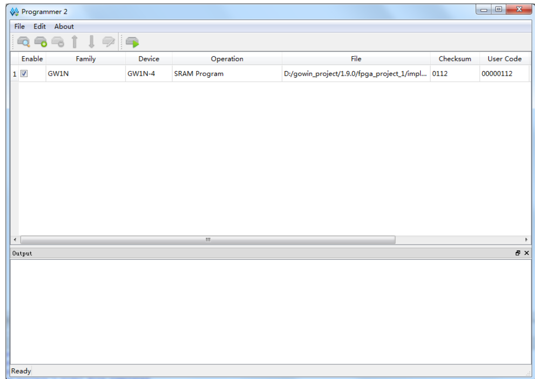
图 5-41 Programmer 界面
