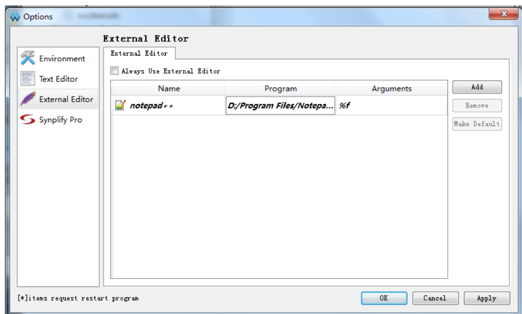
图 5-20 外部编辑器
