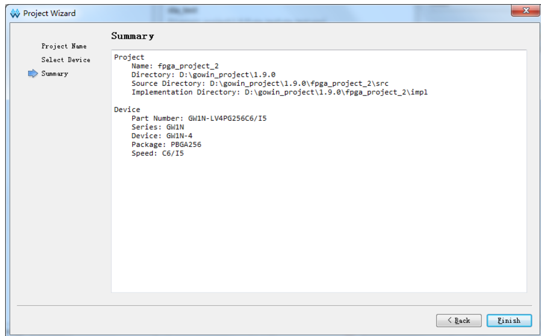
图 5-4 工程信息
