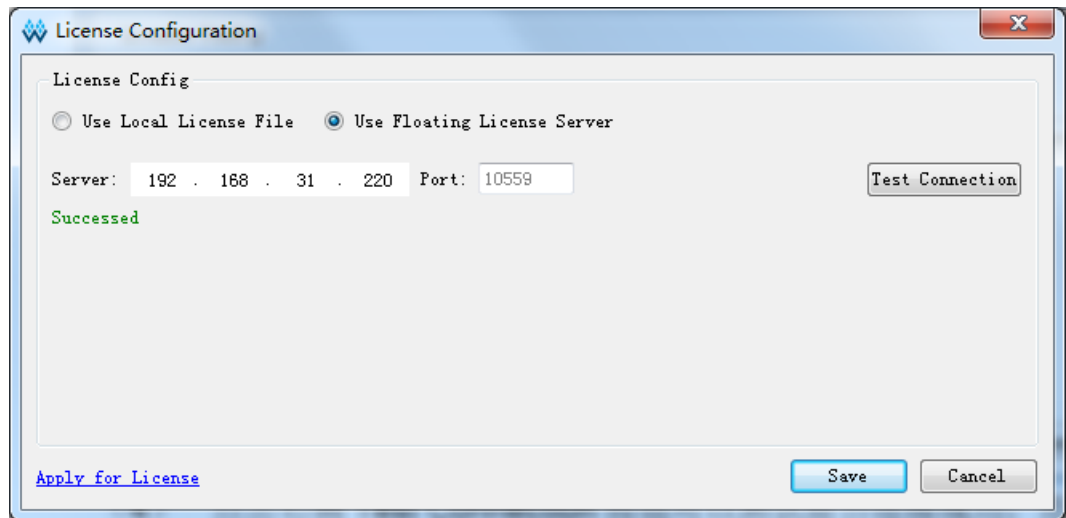
图 3-7 测试连接
