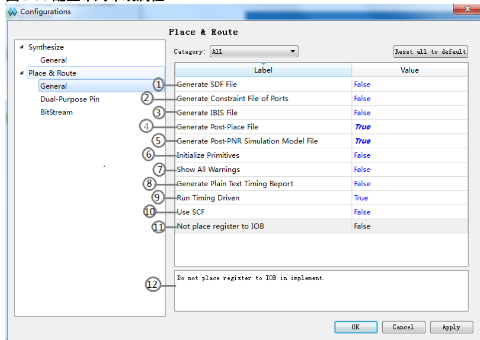
图 5-30 配置布局布线属性
