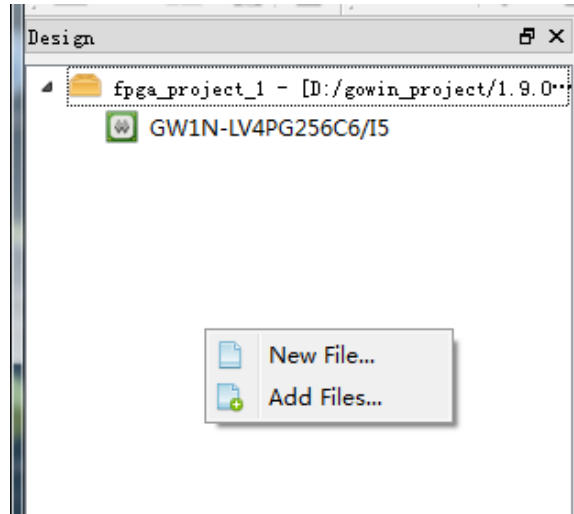
图 5-9 右键菜单
