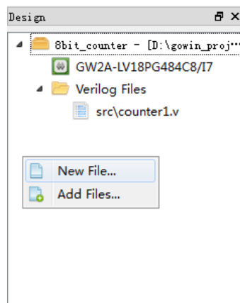
图 4-8 右键菜单
