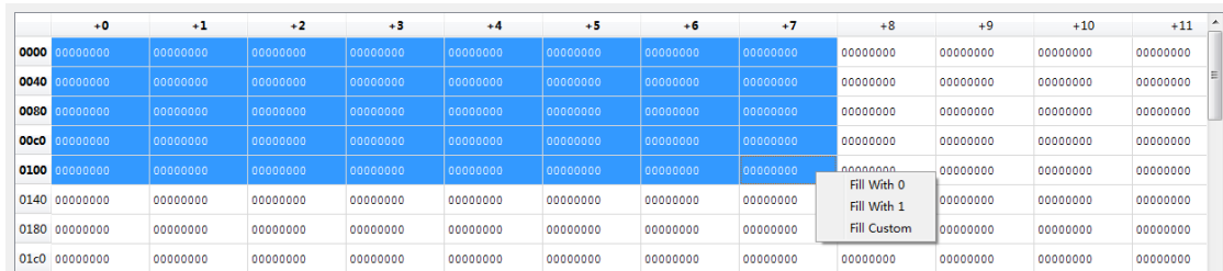
图 5-16 批量设置
