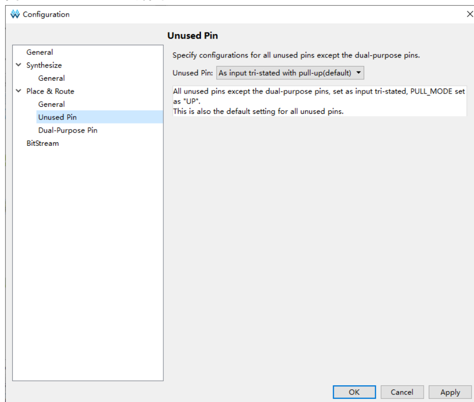
图 4-23 Unused Pin 属性配置
