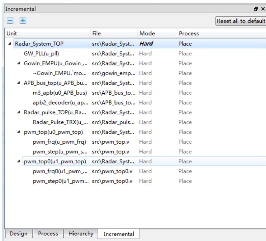
图 4-34 增量编译配置界面
