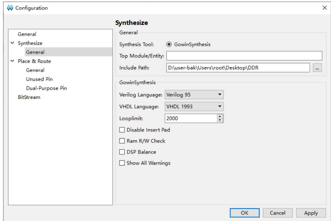
图 4-21 GowinSynthesis 参数配置项
