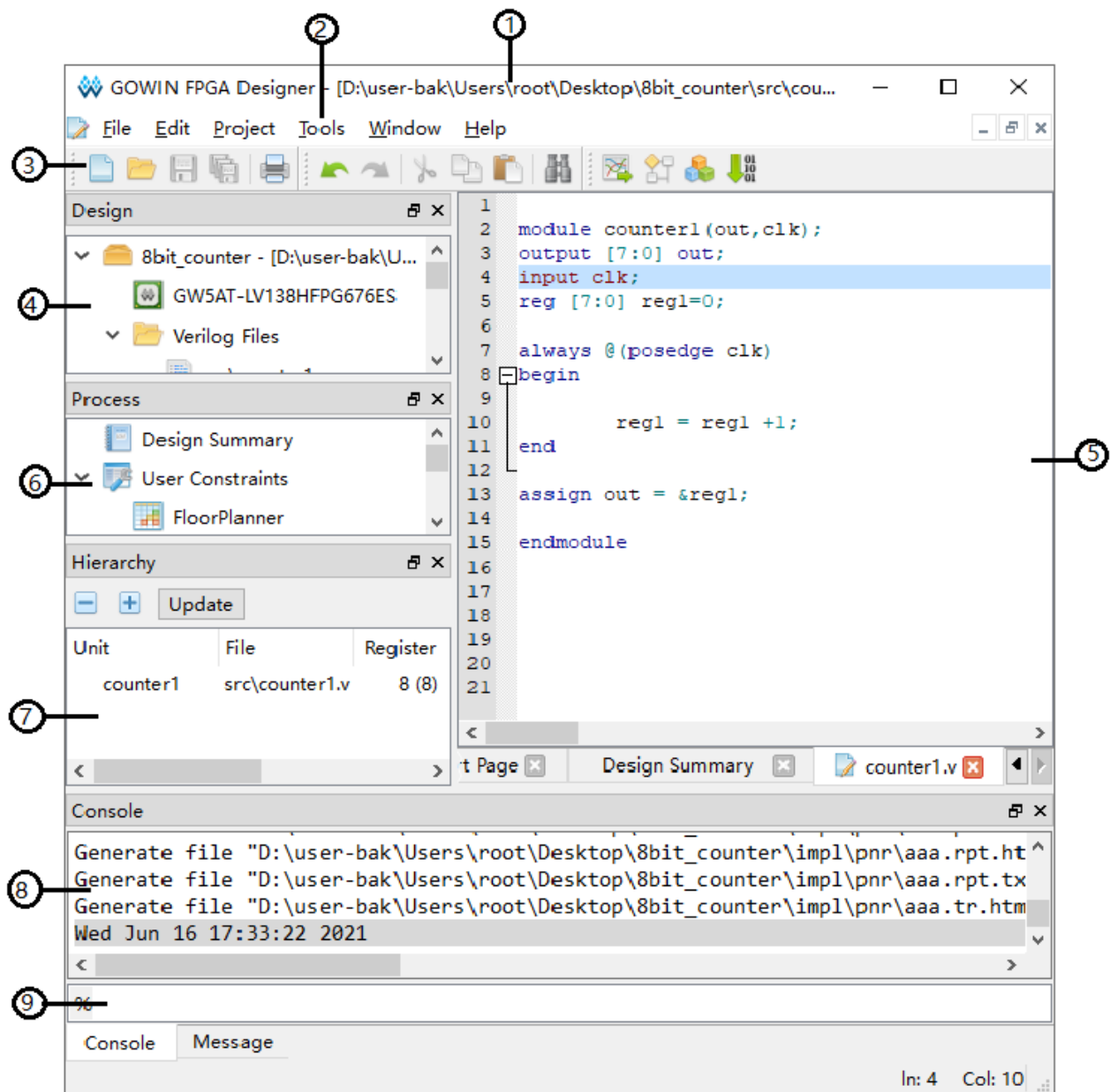
图 3-1 软件用户界面
