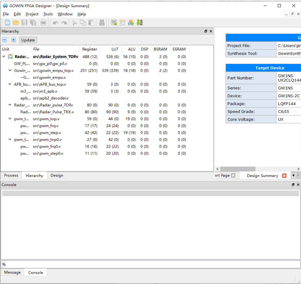
图 3-3 Hierarchy 窗口资源信息显示
