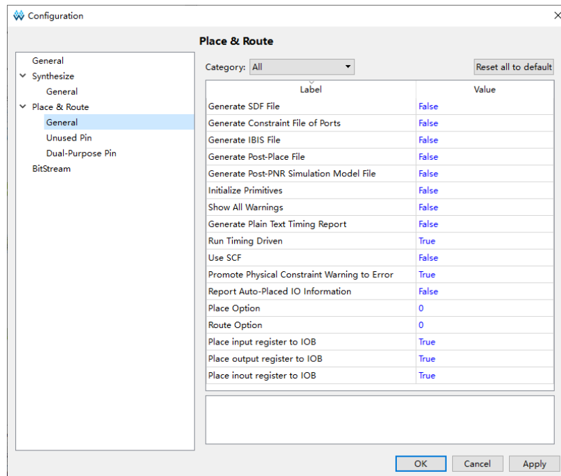
图 4-22 配置布局布线属性
