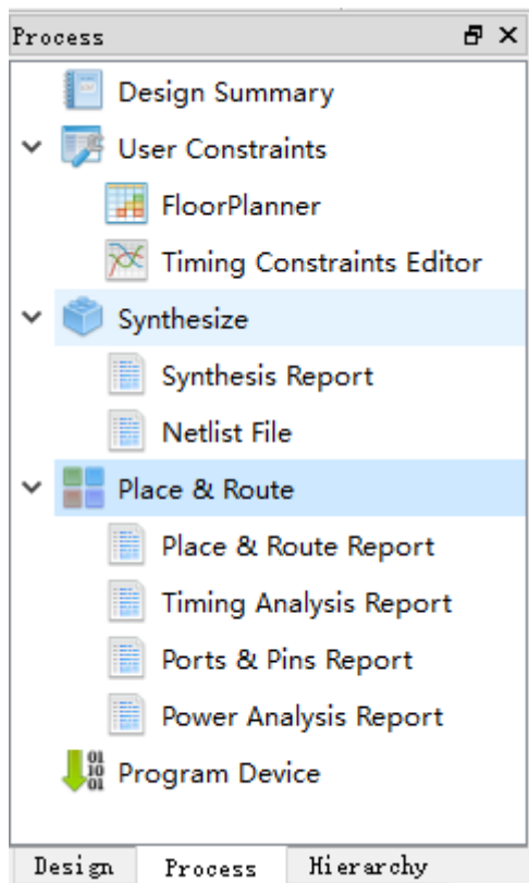
图 4-28 工程 Process 窗口
