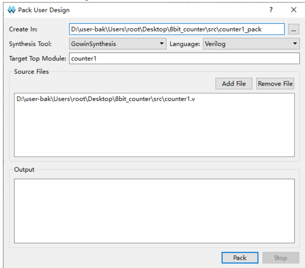
图 3-4 Pack User Design 窗口
