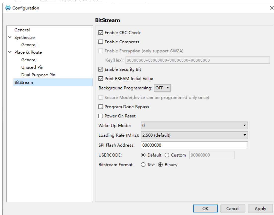
图 4-25 配置比特流文件属性
