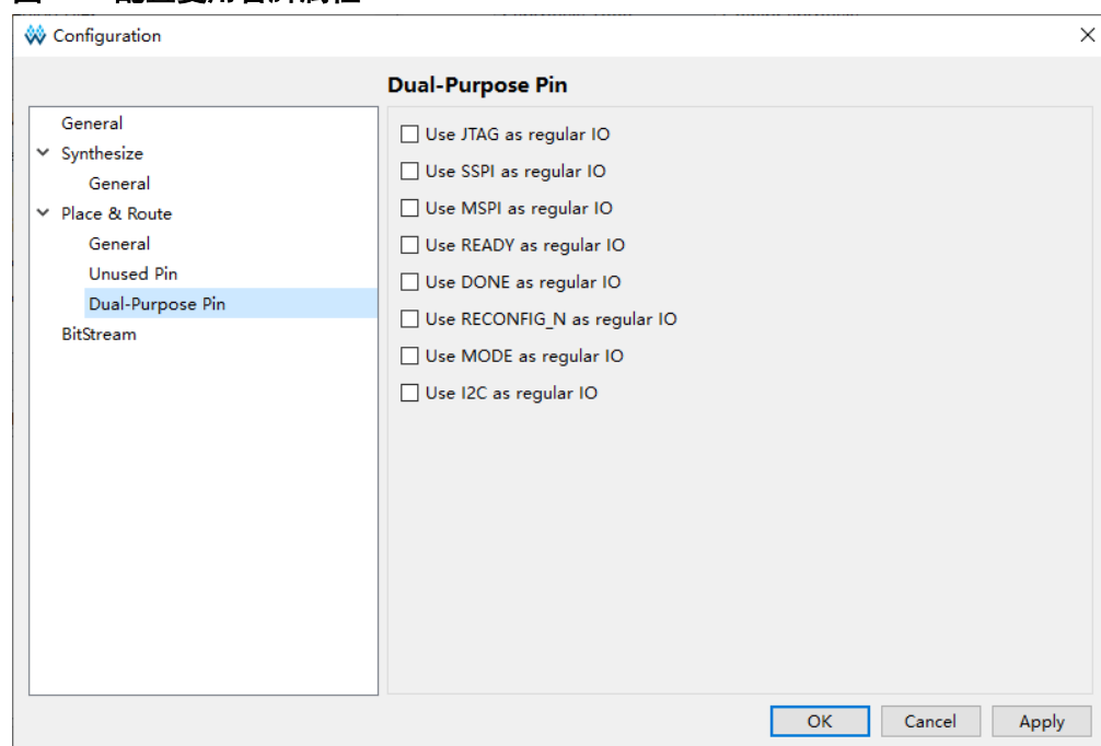
图 4-24 配置复用管脚属性
