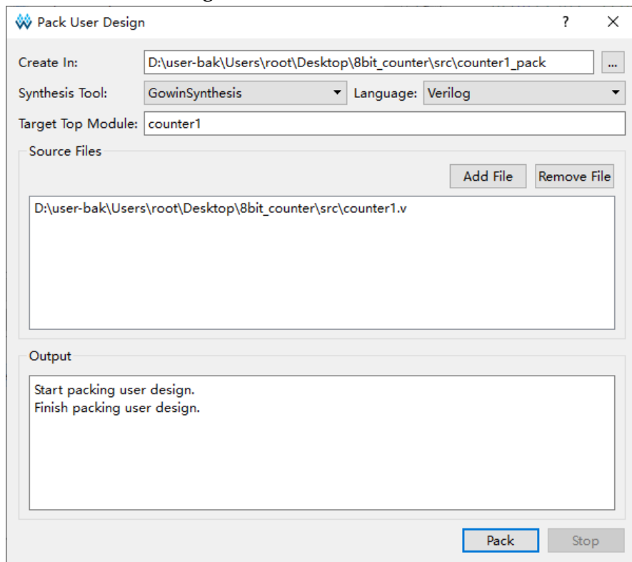
图 3-5 Pack User Design 窗口打印信息
