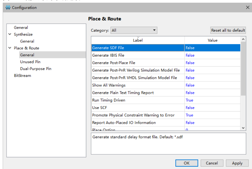
图 4-21 配置布局布线选项
