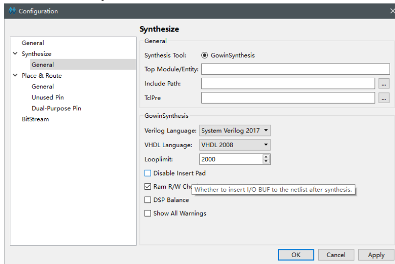
图 4-20 GowinSynthesis 参数配置项
