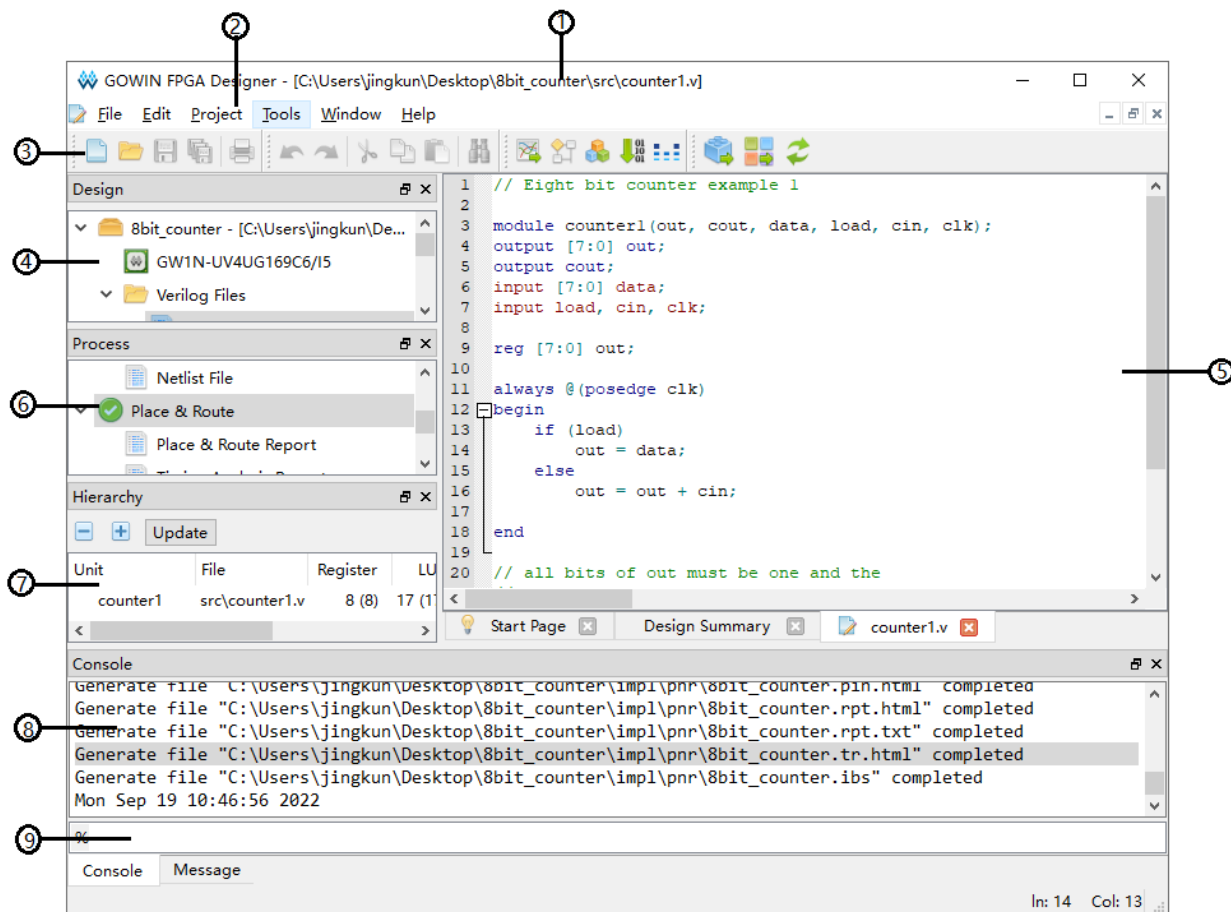
图 3-1 软件用户界面
