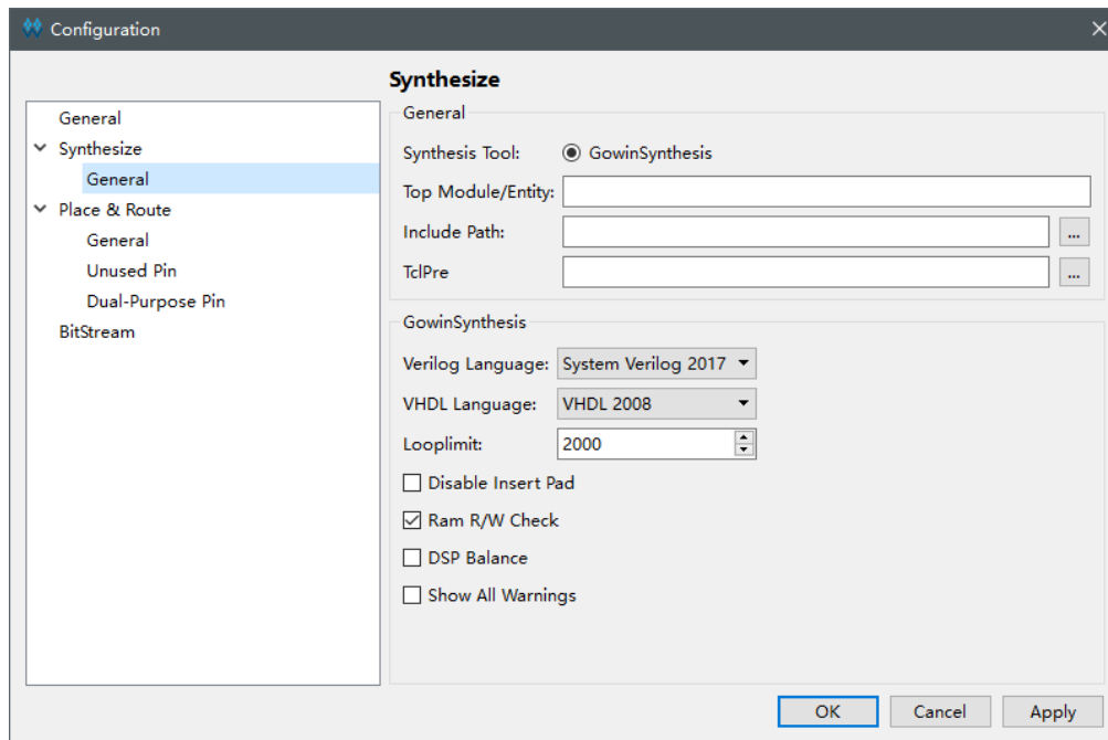
图 4-19 工程配置选项对话框
