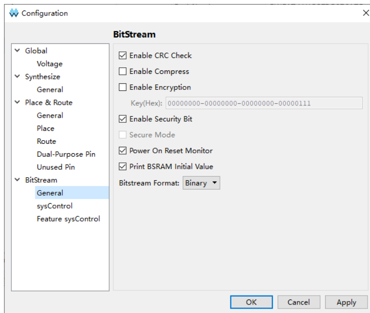
图 4-25 配置 Bitstream General 选项
