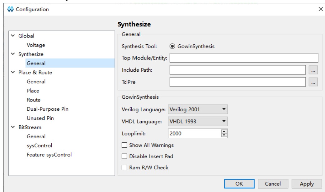
图 4-19 GowinSynthesis 参数配置项
