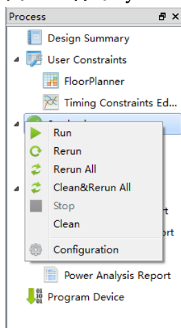
图 4-36 右击 Synthesize
