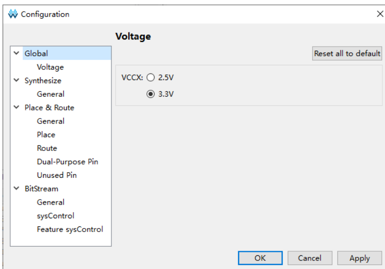
图 4-18 Global 配置项
