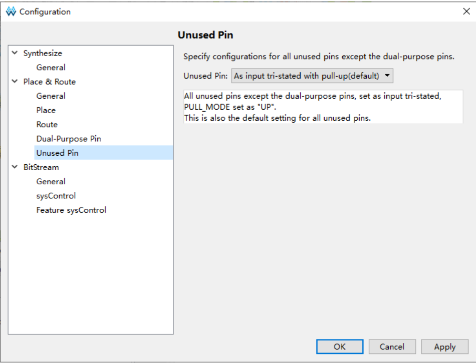
图 4-24 Unused Pin 选项
