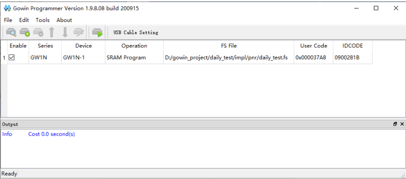
图 4-37 Programmer 界面
