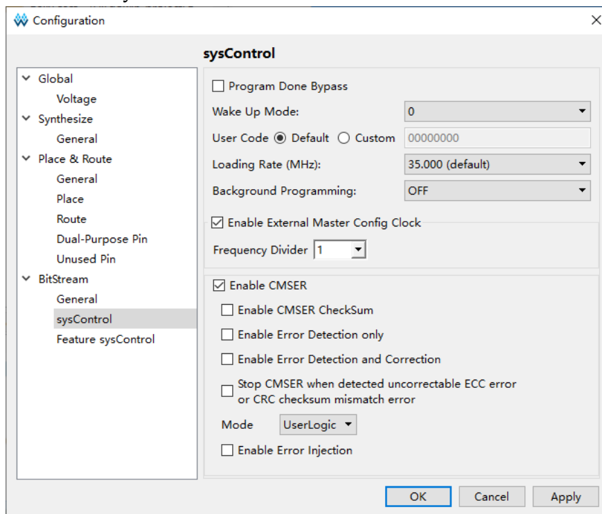
图 4-26 配置 sysControl 选项
