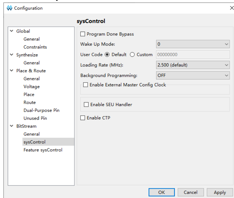
图 4-28 配置 sysControl 选项
