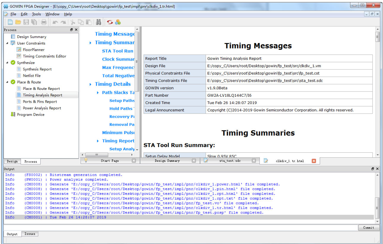
图 4-41 查看时序报告界面
