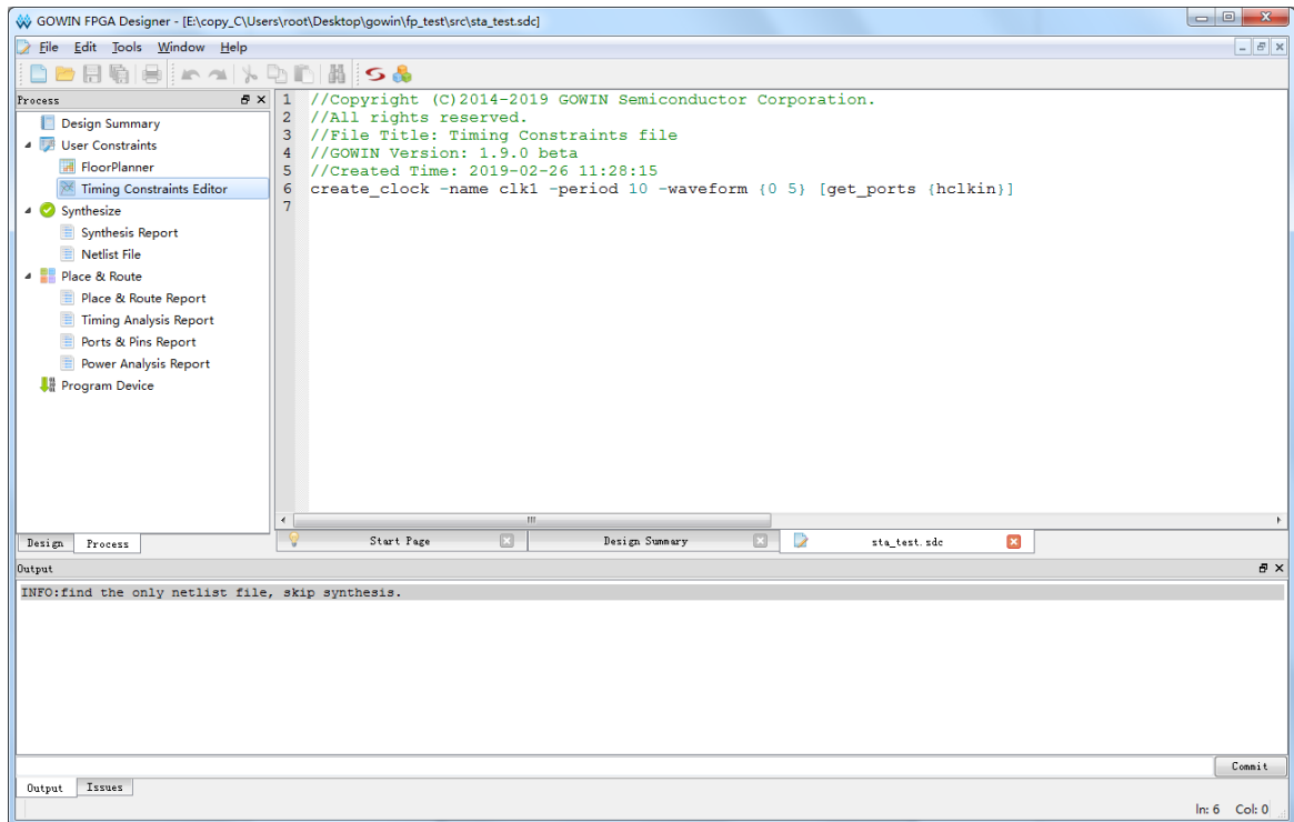
图 4-12 编辑 SDC 文件
