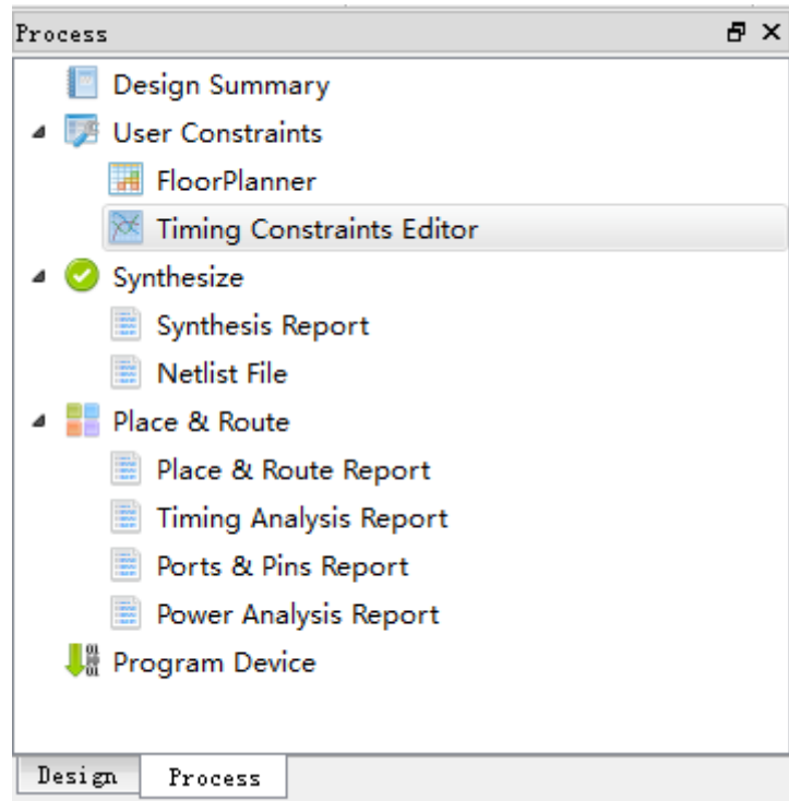
图 4-3 Process 窗口
