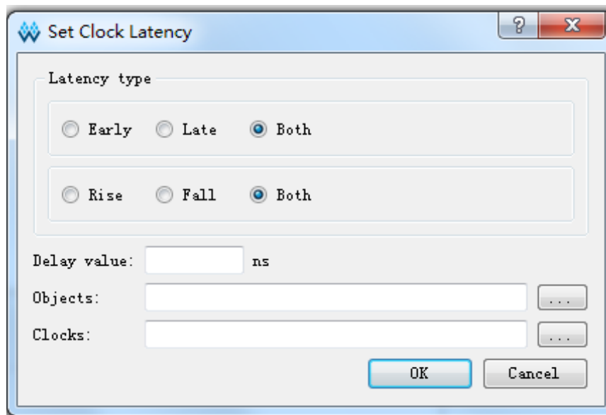
图 4-20 创建 Clock Latency 约束
