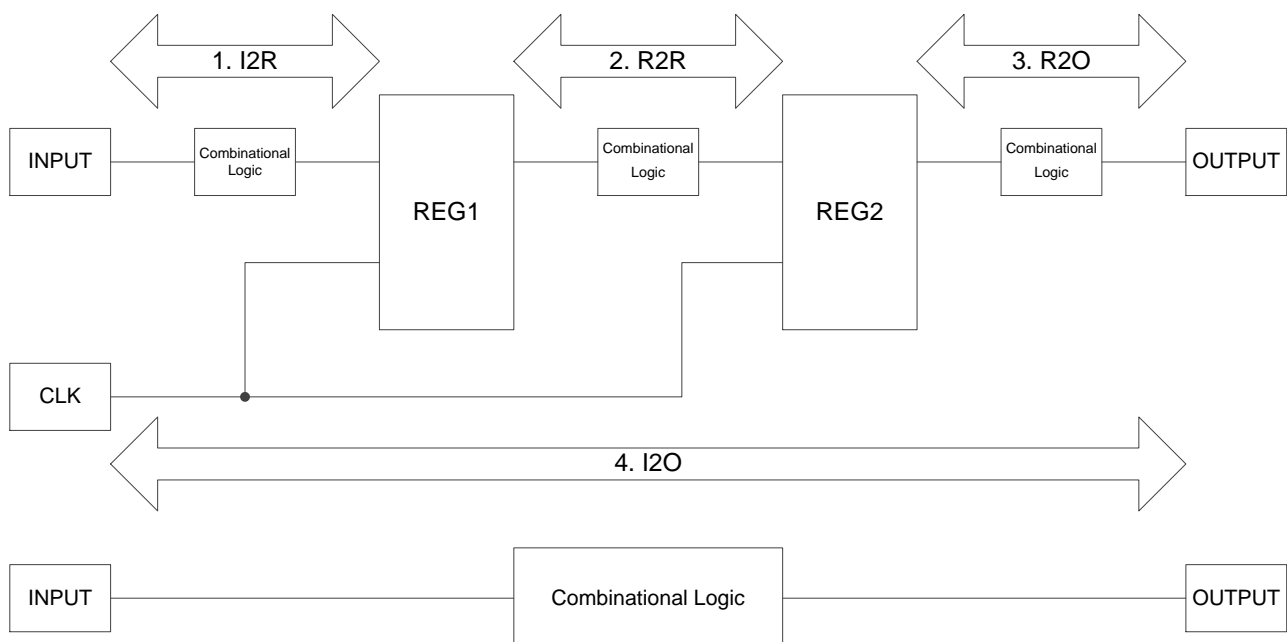
图 4-2 STA 四类时序路径
