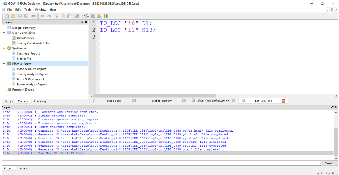
图 3-5 手写物理约束文件
