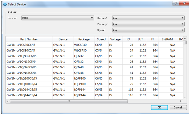
图 3-11 选择器件
