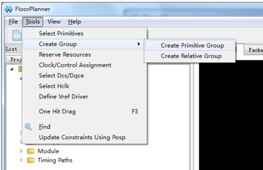
图 3-12 Tools 菜单
