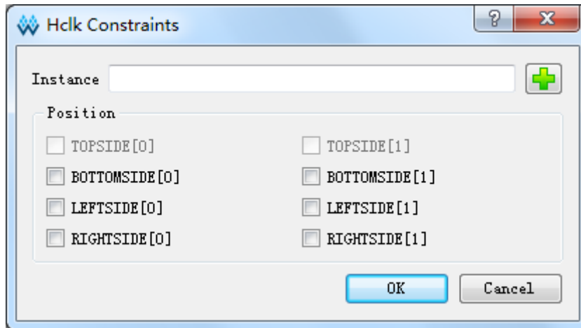
图 3-24 Hclk 约束
