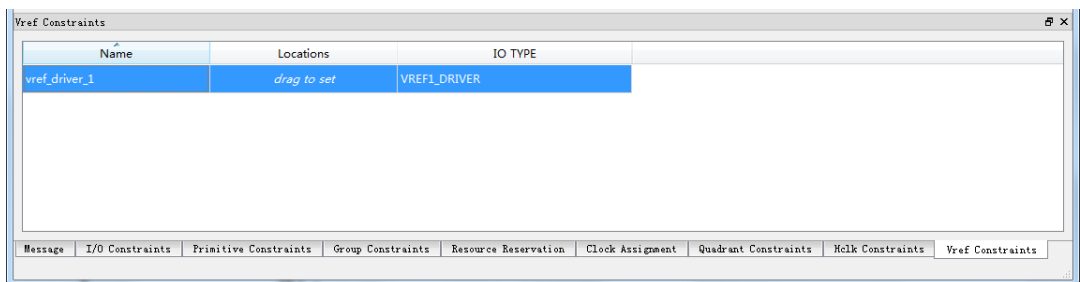
图 3-25 Vref 约束
