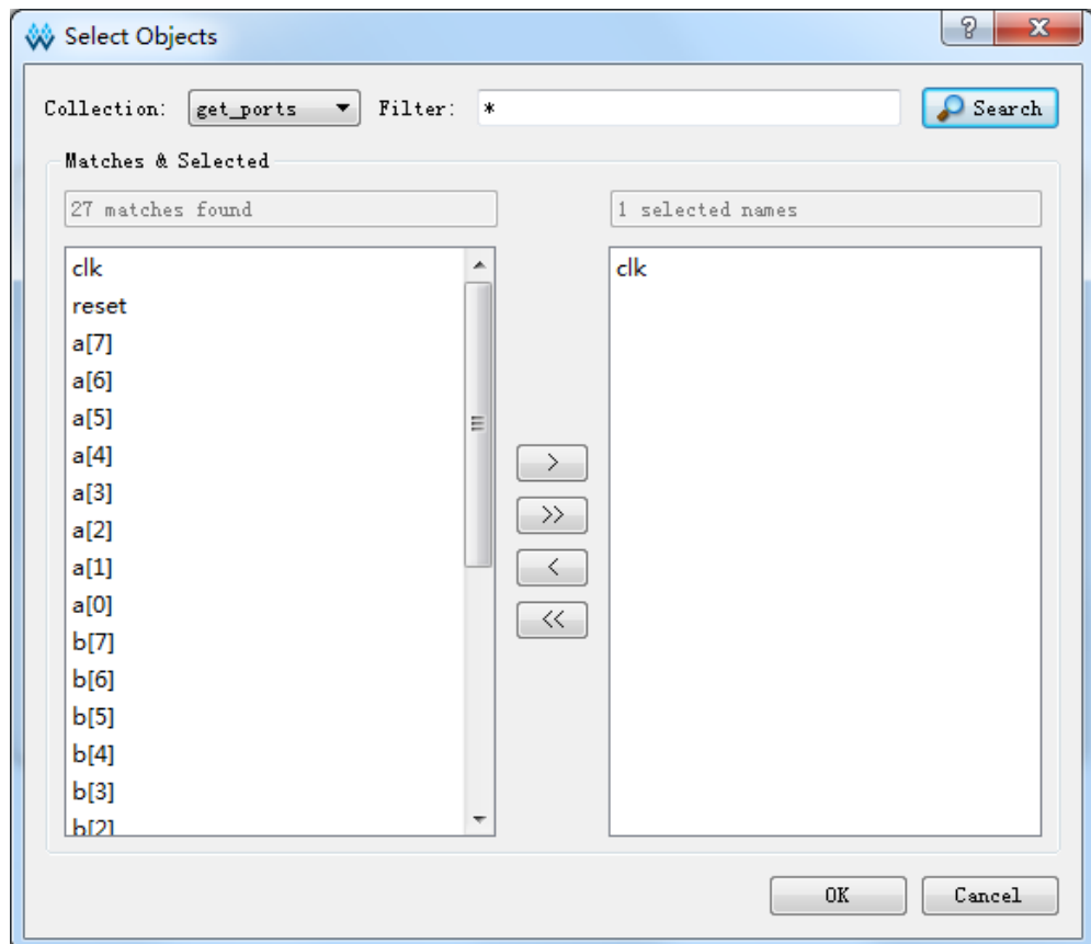
图 4-14 Objects 列表
