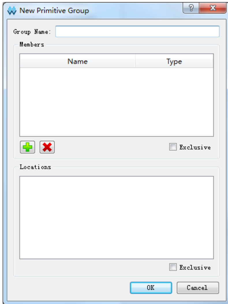
图 3-14 新建原语组
