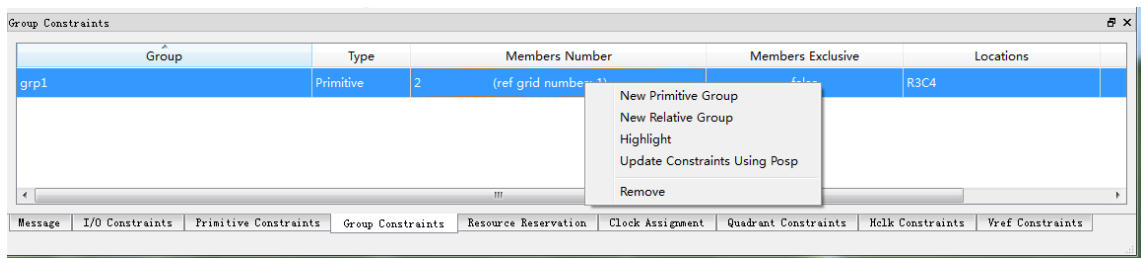
图 3-51 组约束窗口
