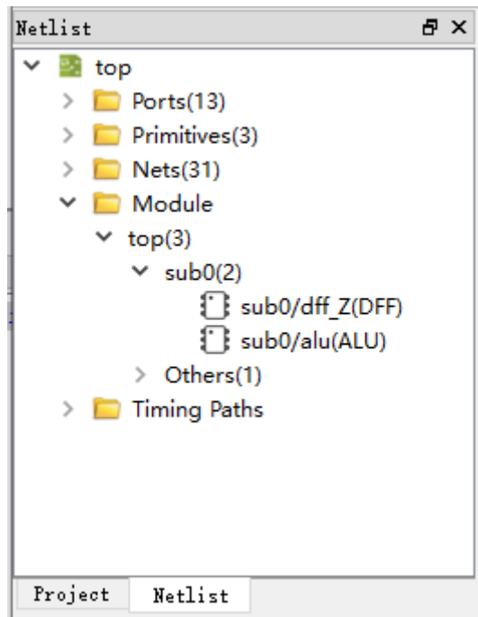
图 3-36 层级显示
