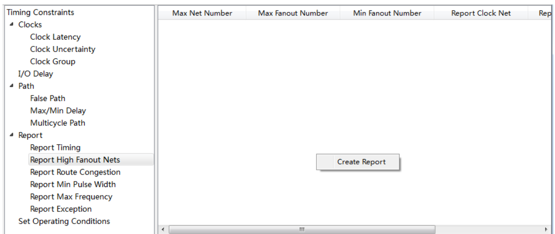
图 4-31 Report High Fanout Nets 创建界面
