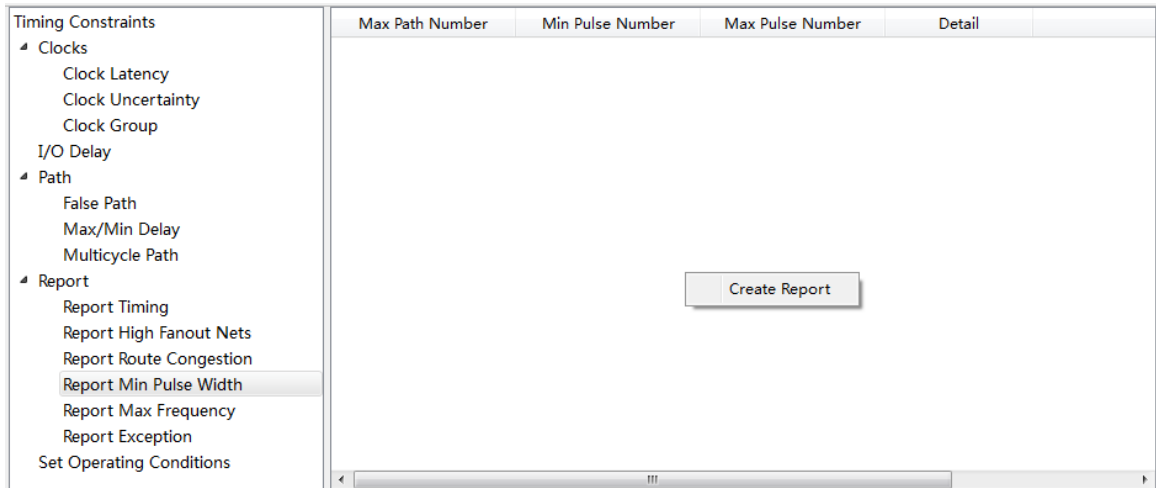
图 4-35 Report Min Pulse Width 创建界面
