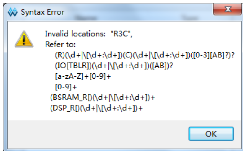
图 3-16 无效位置
