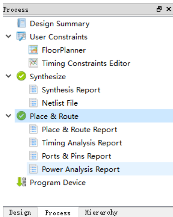
图 4-3 Process 窗口
