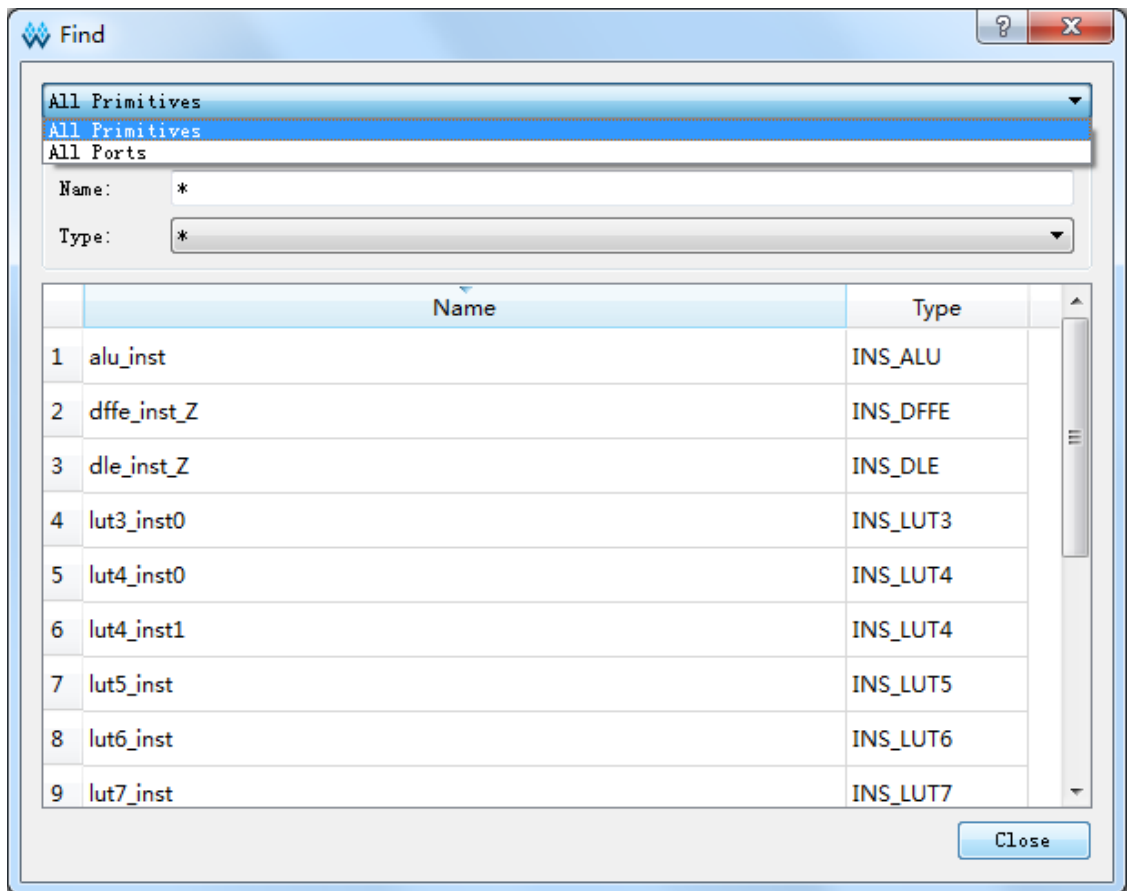
图 3-29 查找界面
