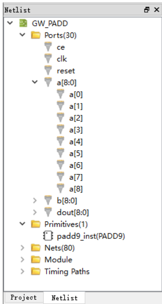
图 3-34 Netlist 窗口
