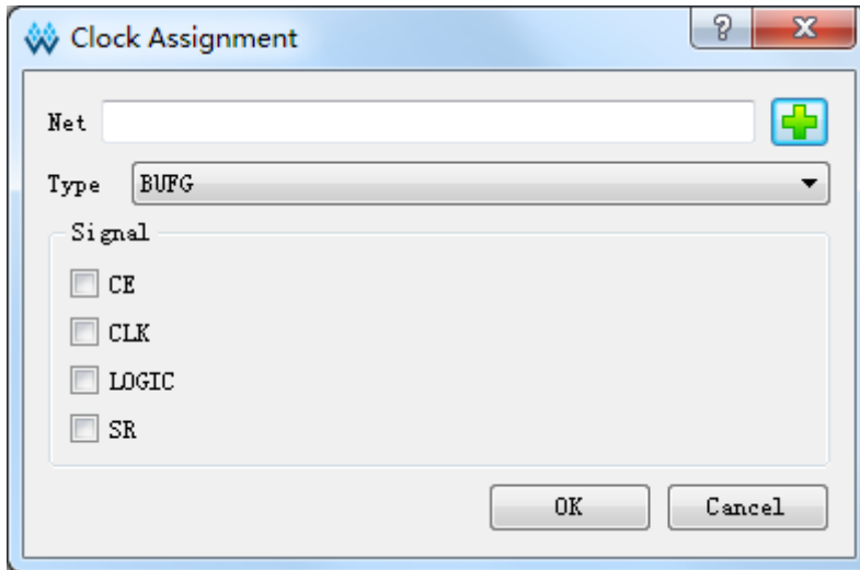
图 3-21 时钟约束
