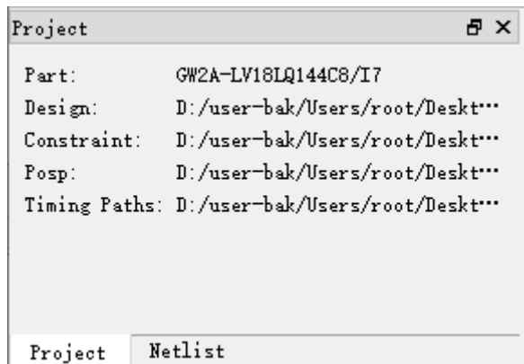
图 3-33 Project 窗口
