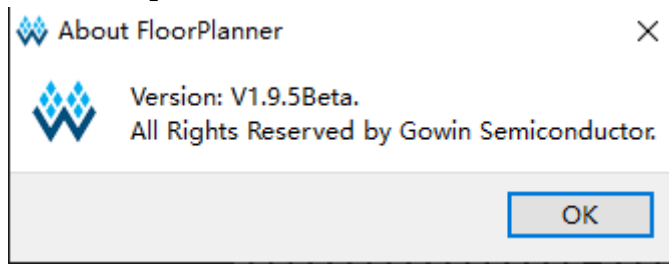
图 3-32 Help 提示框
