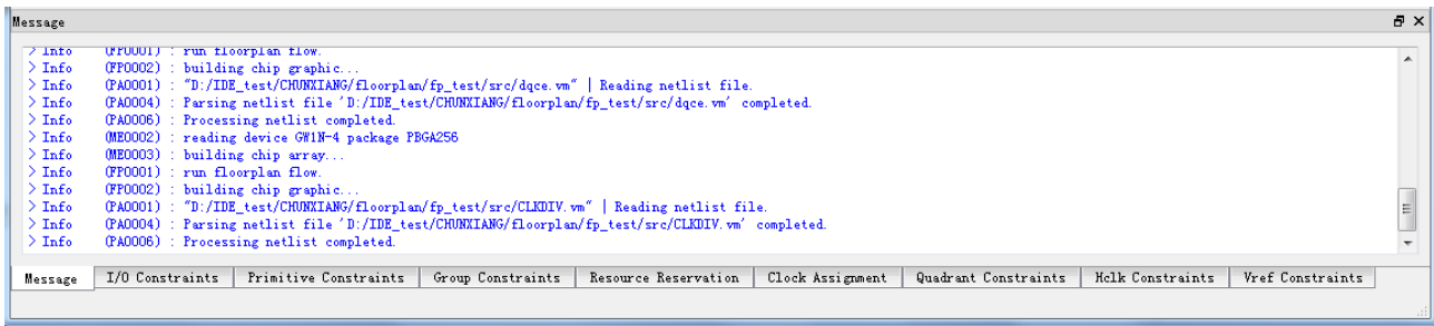
图 3-57 Message 窗口
