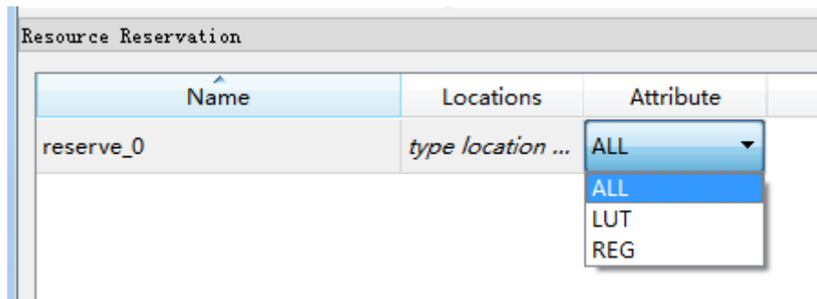
图 3-20 预留约束
