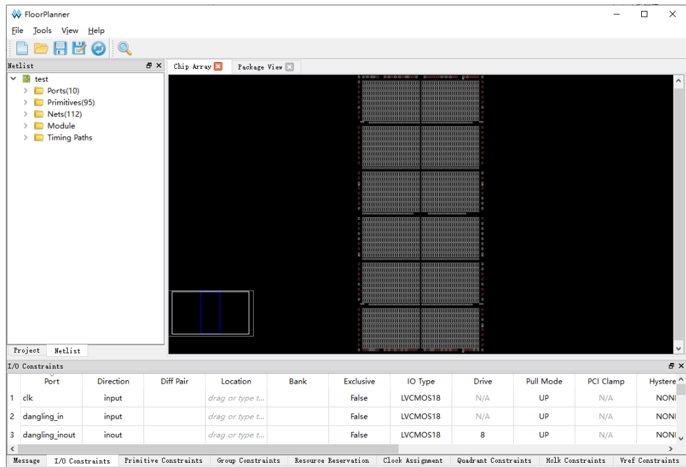
图 3-9 FloorPlanner 界面
