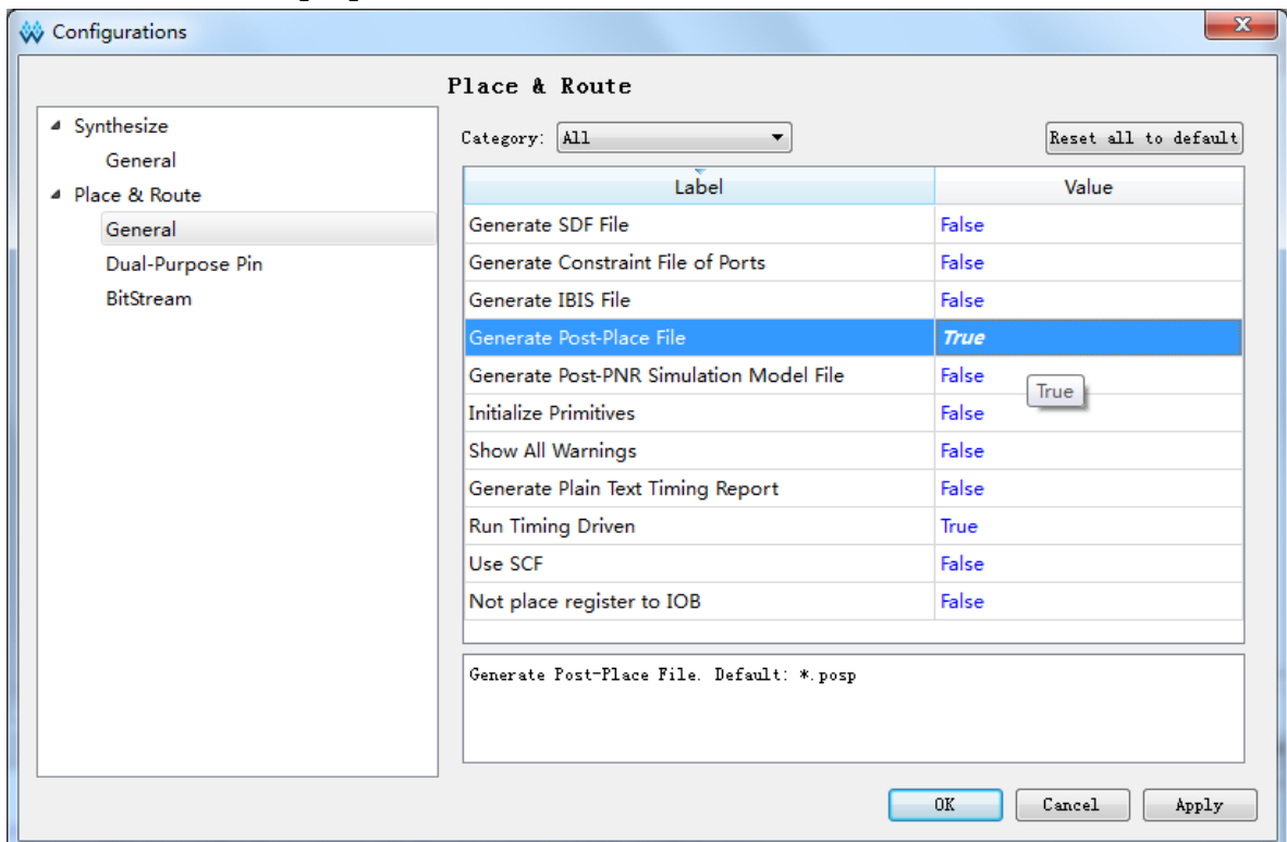
图 5-1 生成 .posp 文件设置
