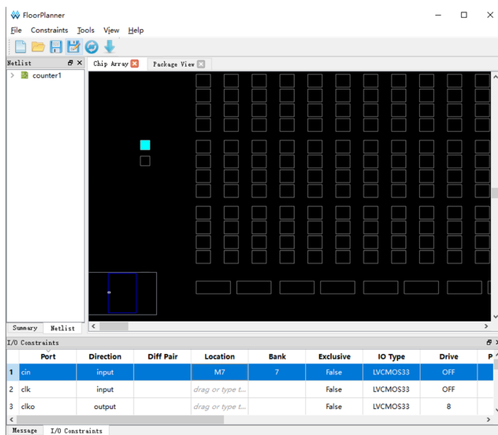
图 4-4 拖拽到 Chip Array 创建 I/O Constraints
