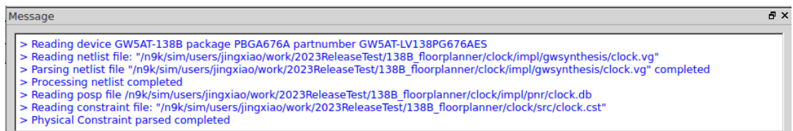
图 3-51 Message 窗口
