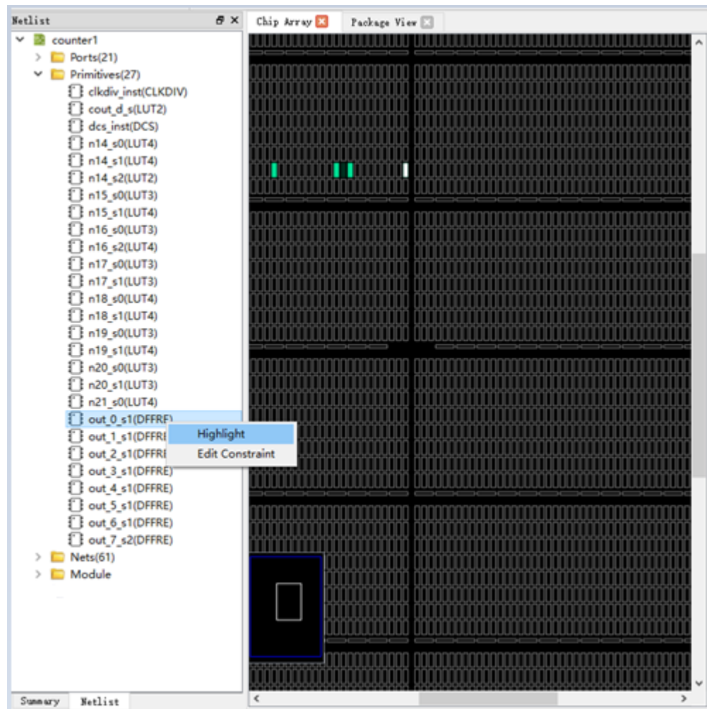
图 3-42 右键高亮
