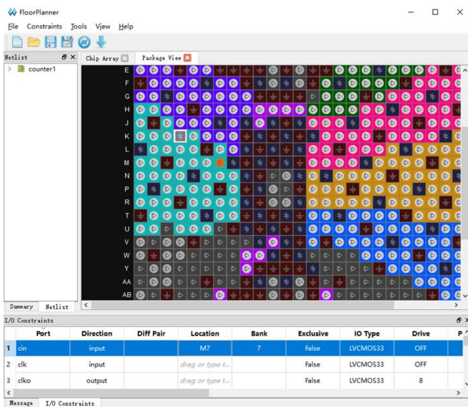
图 4-5 拖至 Package View 创建 I/O Constraints
