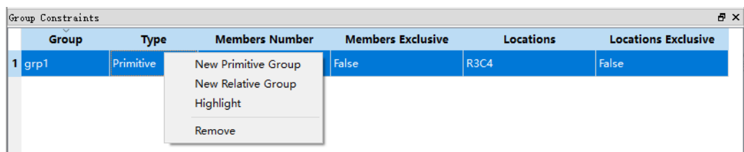
图 3-45 组约束窗口
