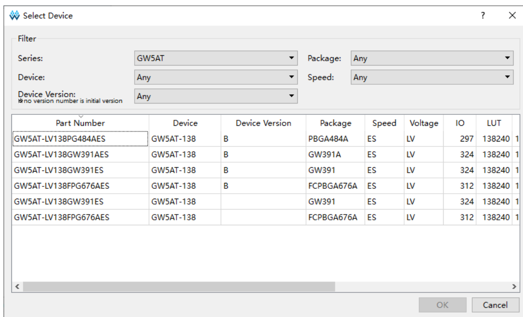
图 4-2 选择器件
