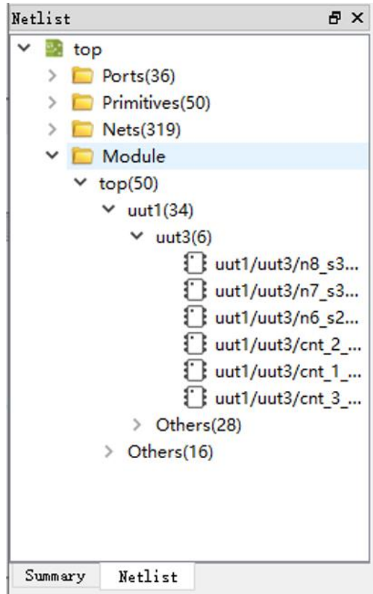
图 3-28 层级显示
