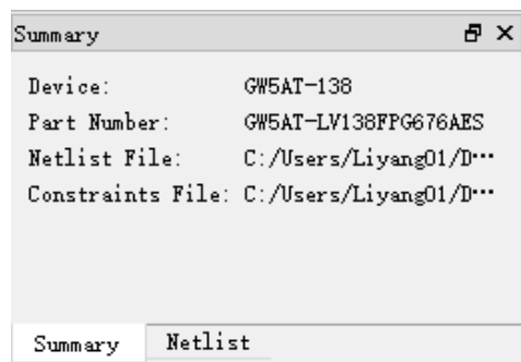
图 3-25 Summary 窗口
