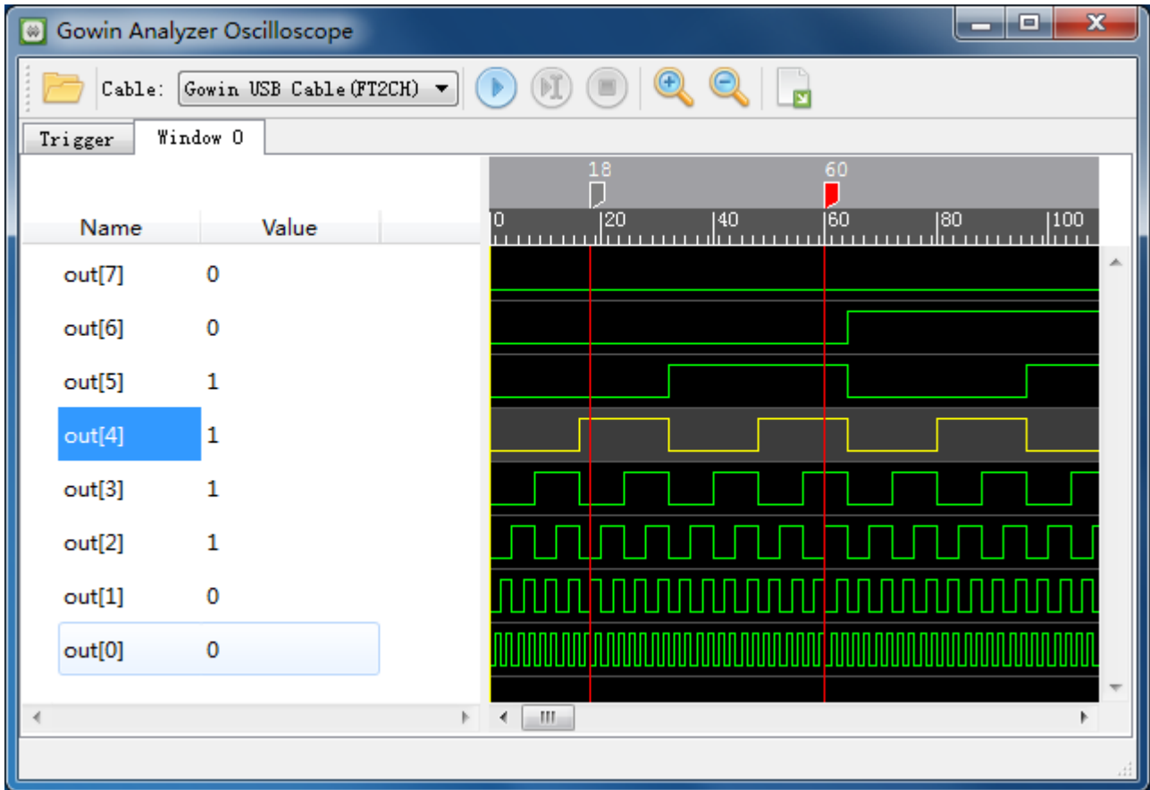
图 4-17 标尺和游标显示 (Lite Mode)
