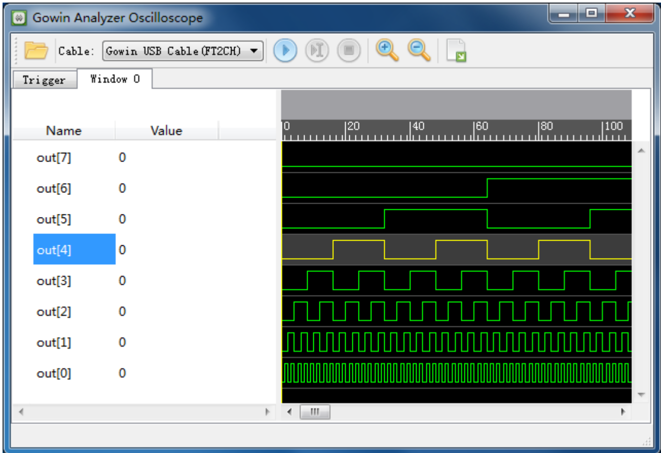
图 4-16 逻辑分析仪波形显示 (Lite Mode)
