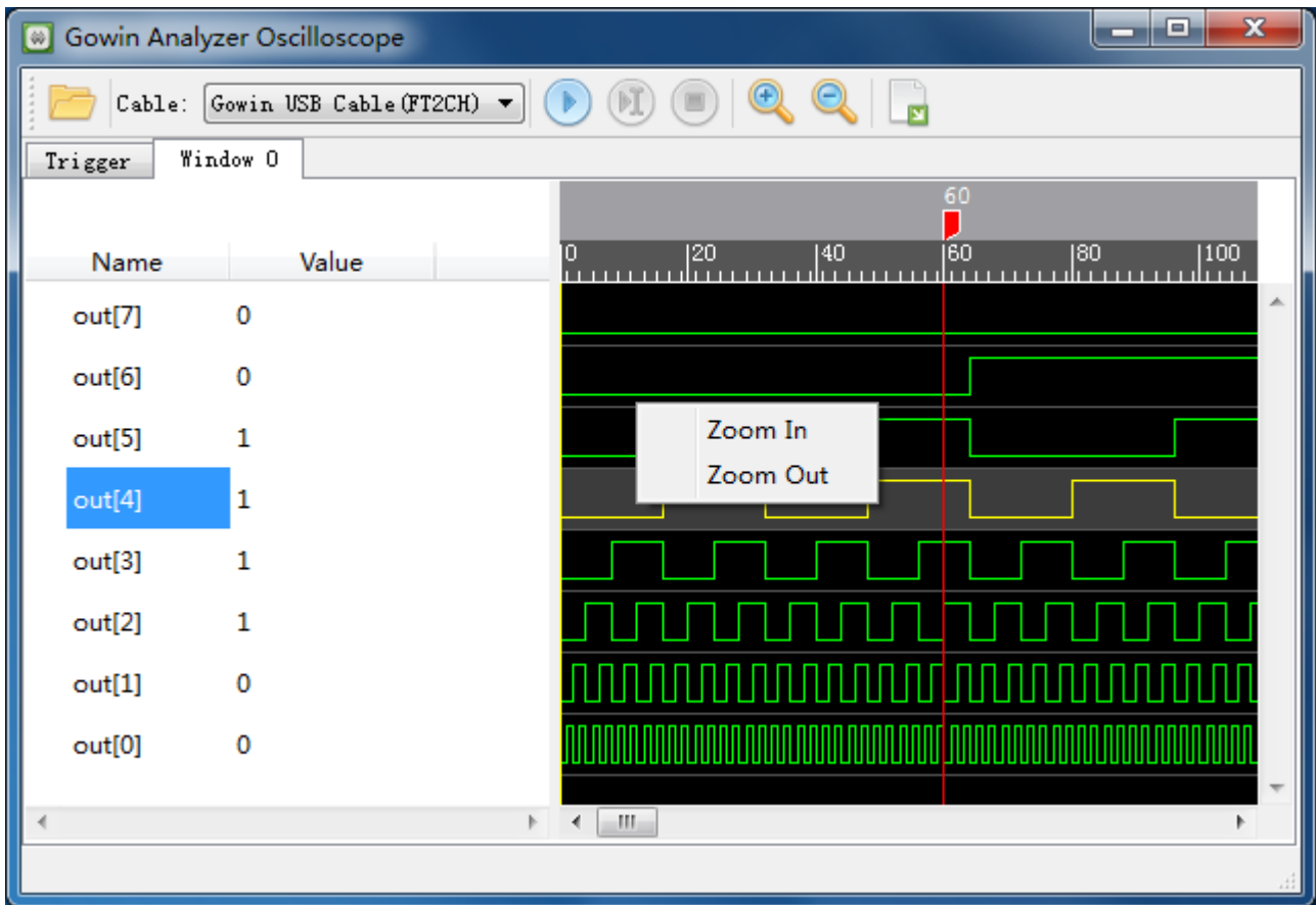
图 4-18 右键放大缩小菜单栏（Lite Mode）
