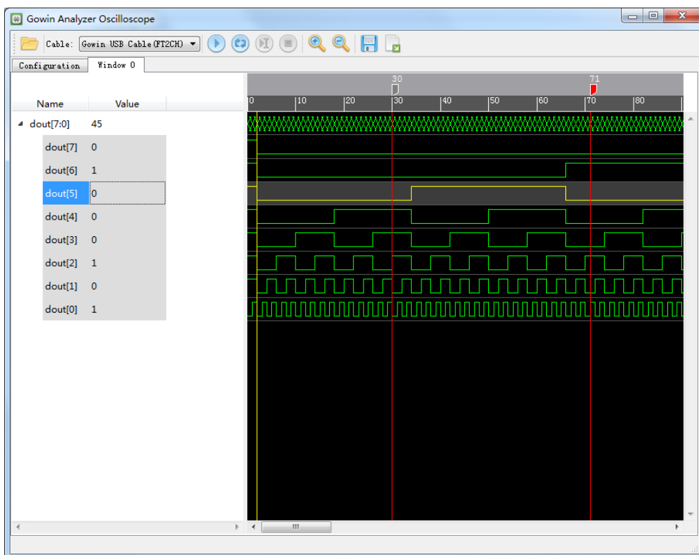
图 4-8 标尺和游标显示 (Standard Mode)
