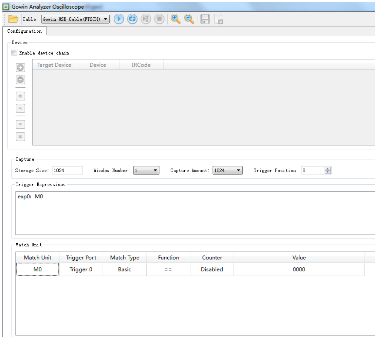
图 4-1 Gowin Analyzer Oscilloscope 工具界面 (Standard Mode)
