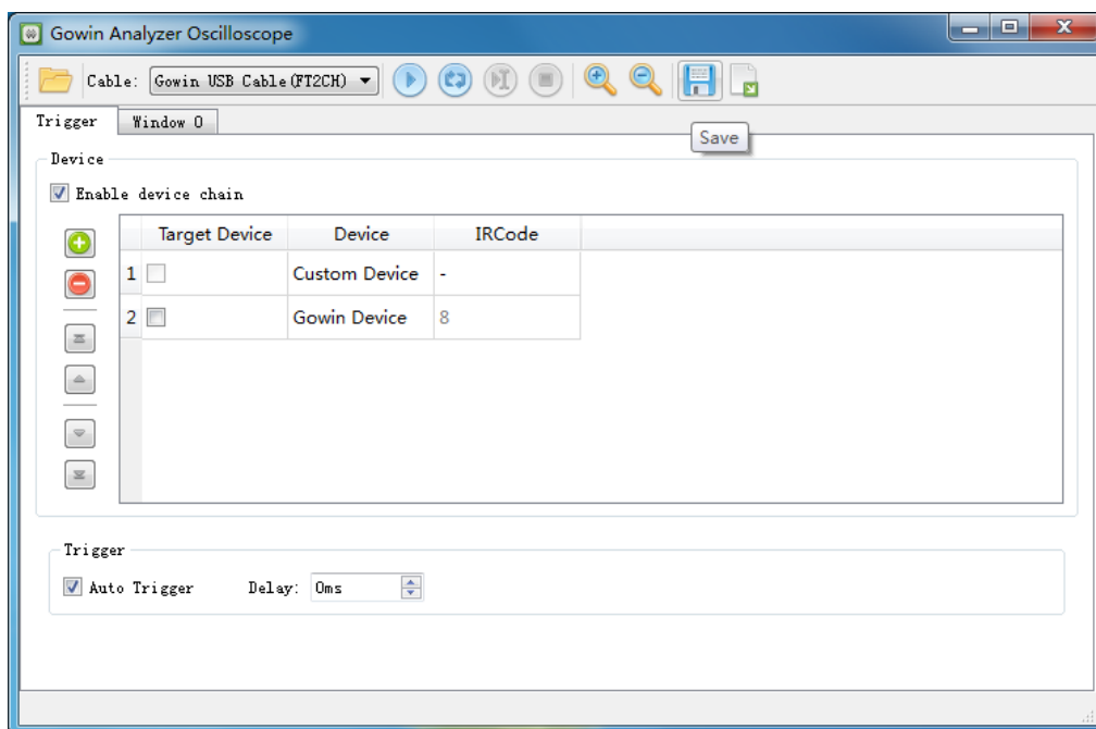
图 4-13 Gowin Analyzer Oscilloscope 工具界面 (Lite Mode)
