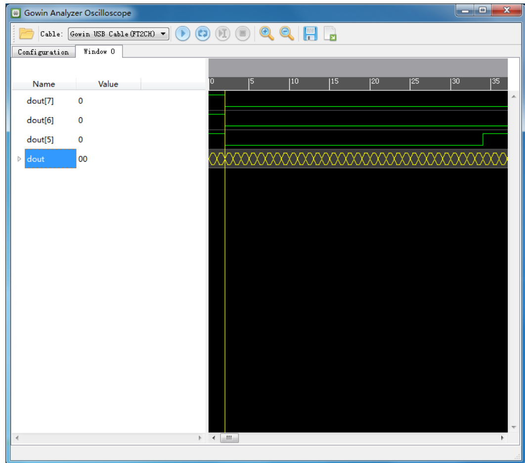
图 4-10 组成 Bus 信号 (Standard Mode)
