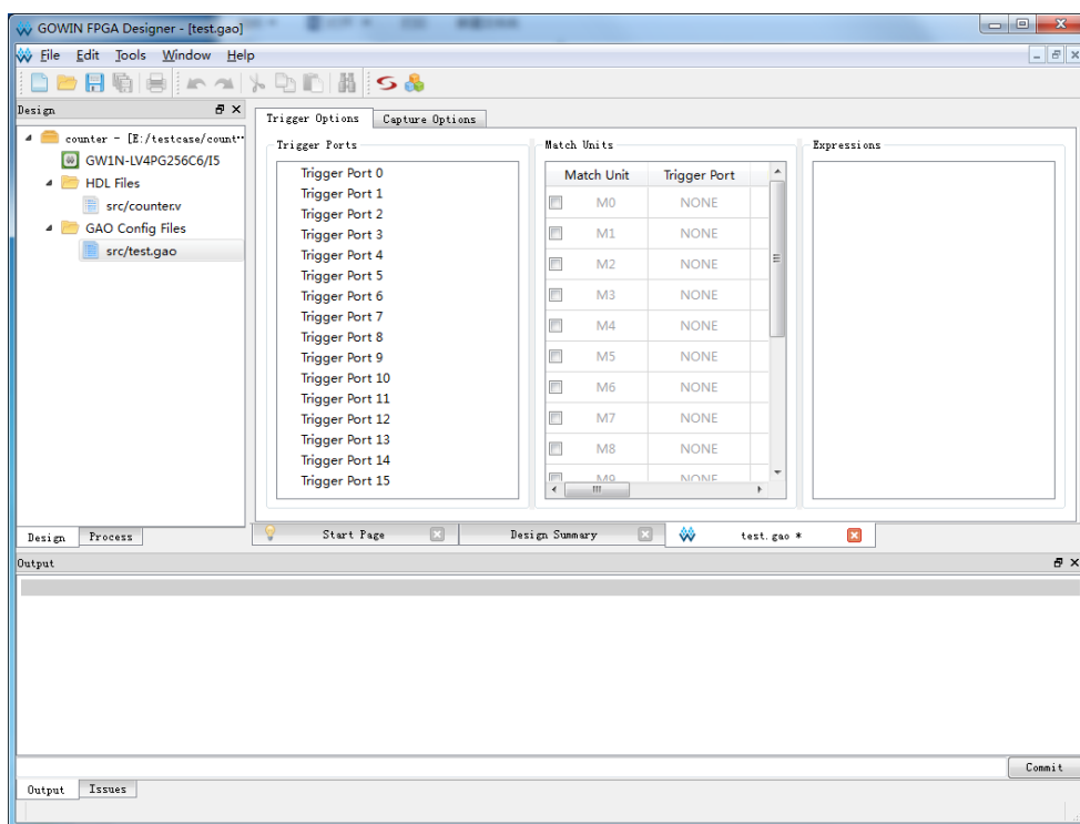
图 3-6 Gowin GAO 配置工具界面 (Standard Mode)
