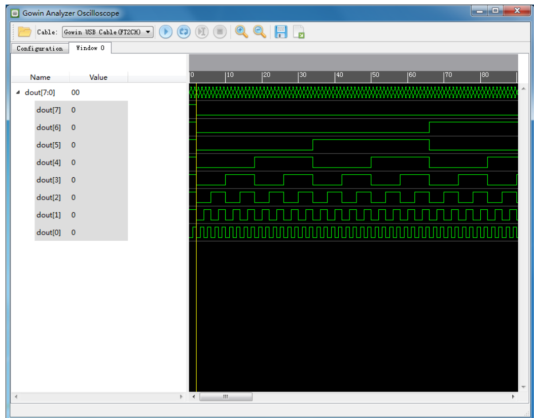
图 4-6 逻辑分析仪波形显示 (Standard Mode)
