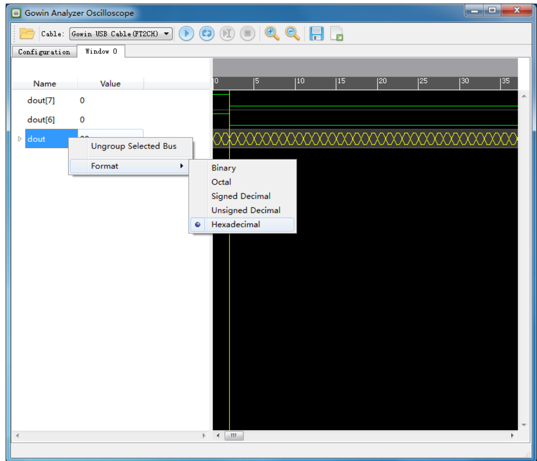
图 4-11 右键进制菜单栏 (Standard Mode)
