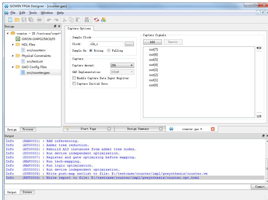
图 3-36 Gowin GAO 配置工具界面 (Lite Mode)
