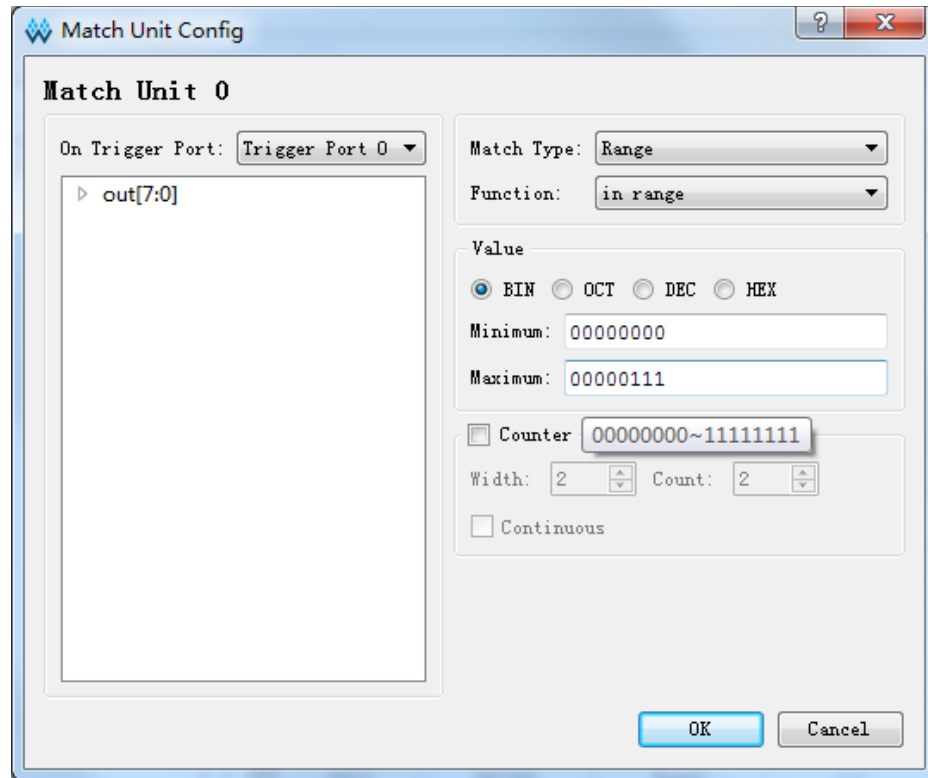
图 3-16 范围内/外检测的 Minimum/Maximum 设置
