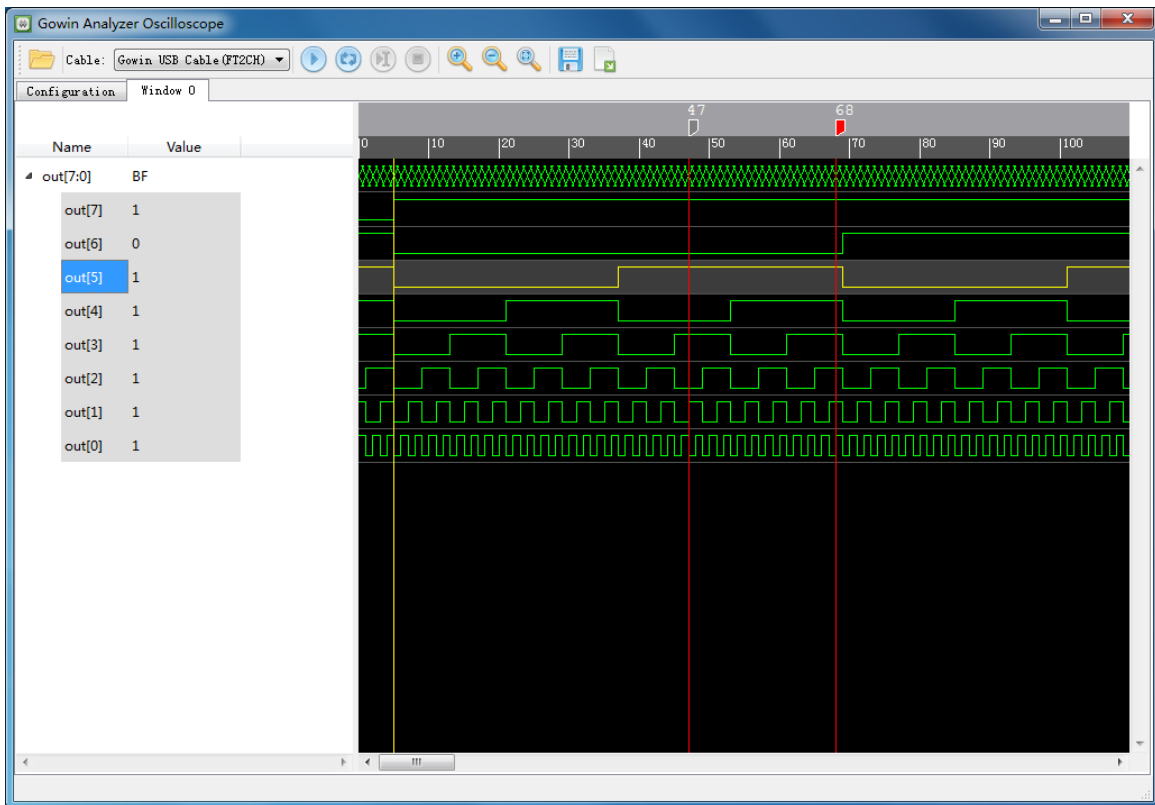
图 4-8 标尺和游标显示 (Standard Mode)
