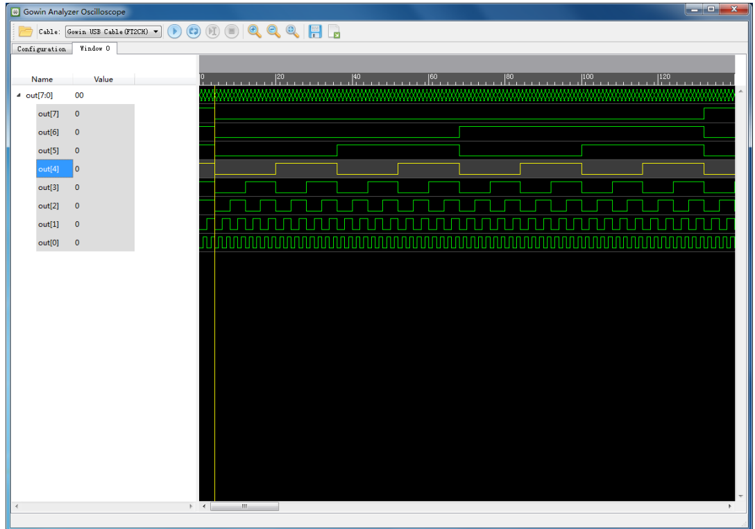
图 4-6 逻辑分析仪波形显示（Standard Mode）
