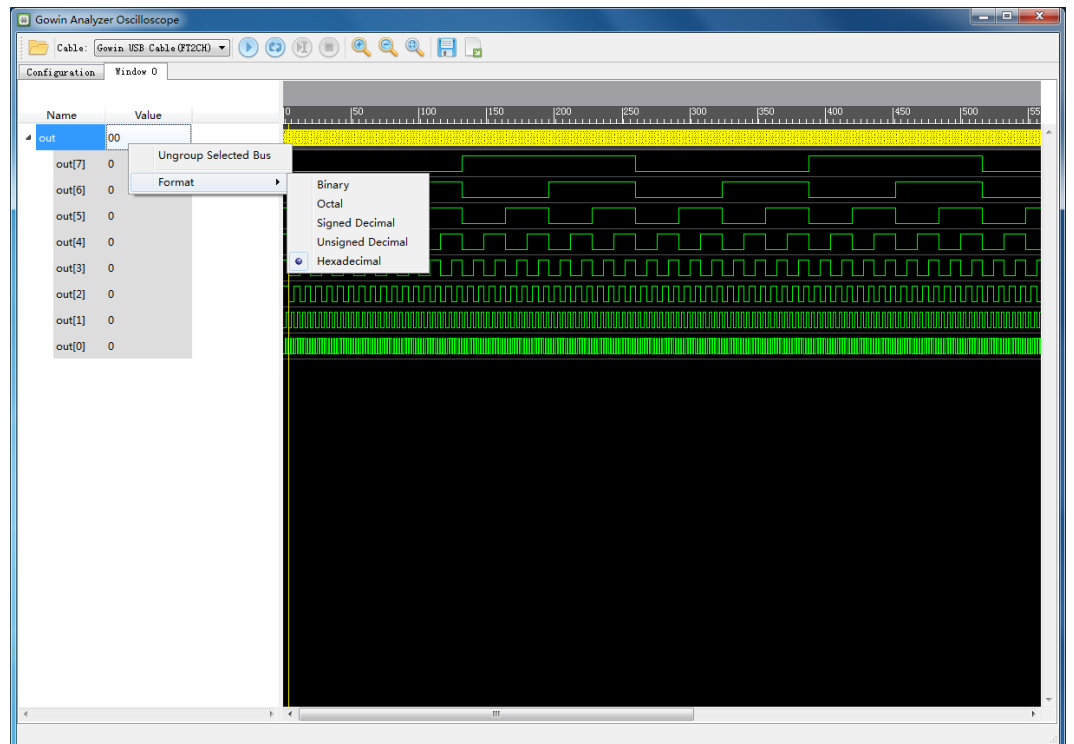
图 4-11 右键进制菜单栏 (Standard Mode)
