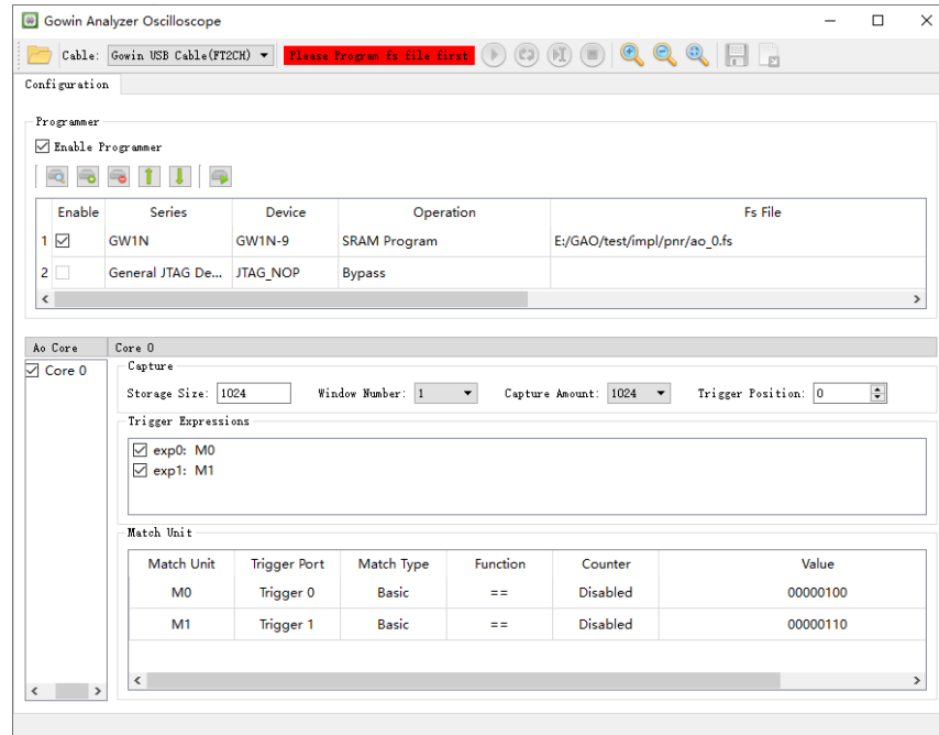
图 4-4 Configuration 窗口
