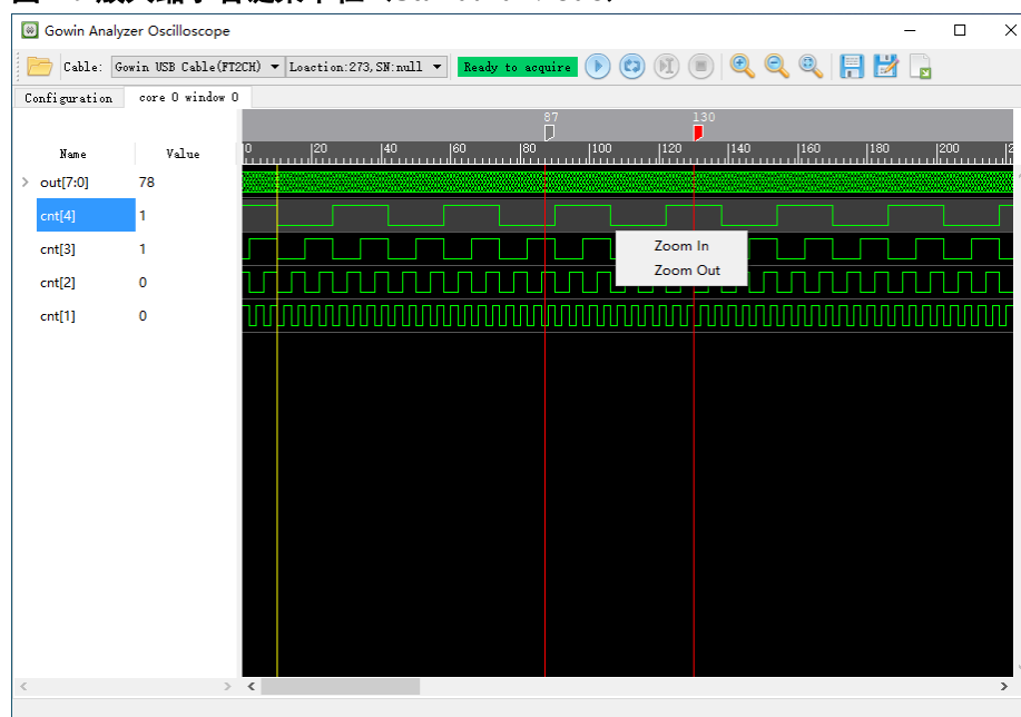
图 4-9 放大缩小右键菜单栏（Standard Mode）
