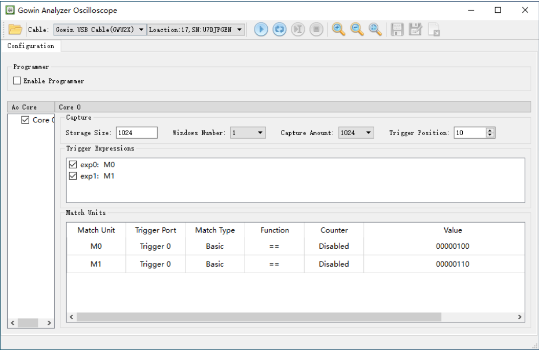
图 4-2 Gowin Analyzer Oscilloscope 工具配置窗口 (Dynamic Standard Mode)
