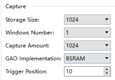
图 3-27 Capture 配置视图
