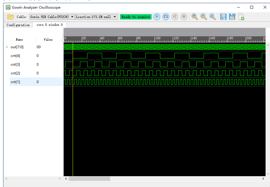
图 4-7 逻辑分析仪波形显示（Standard Mode）
