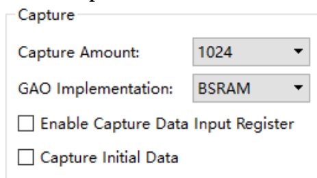
图 3-41 Capture 配置视图（Lite Mode）
